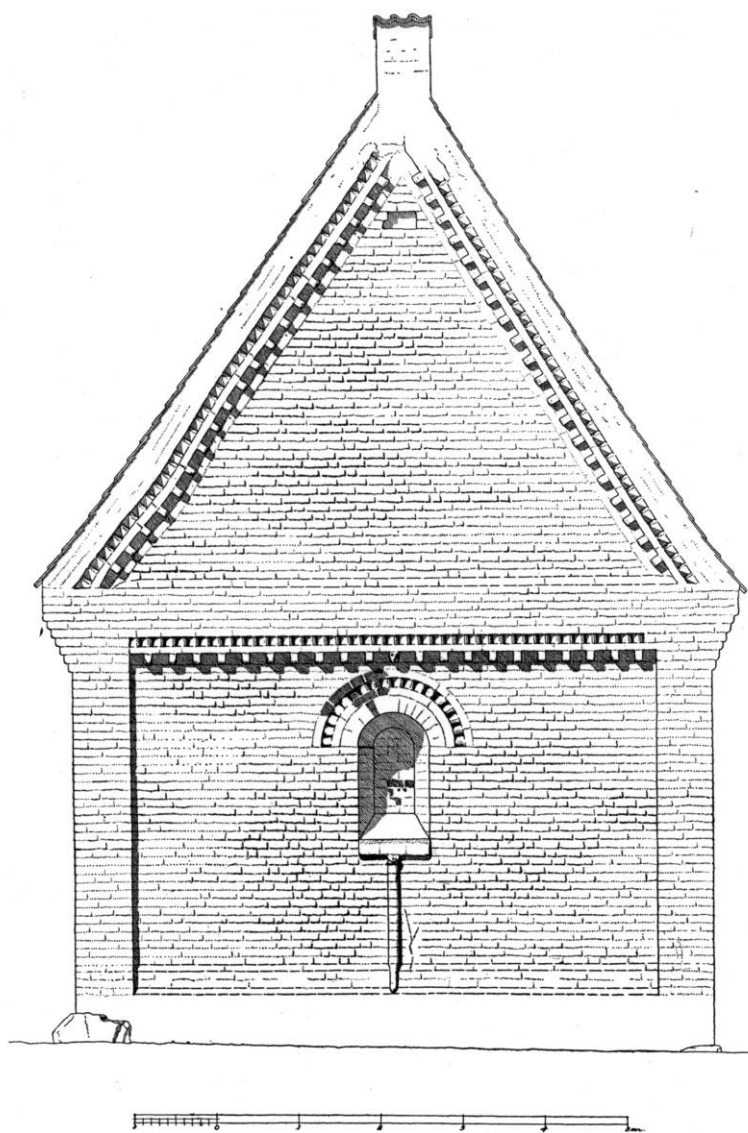
Fig. 3. Aastrup. Korets østgavl. 1:100. Målt af Karl Bisgaard 1943.
