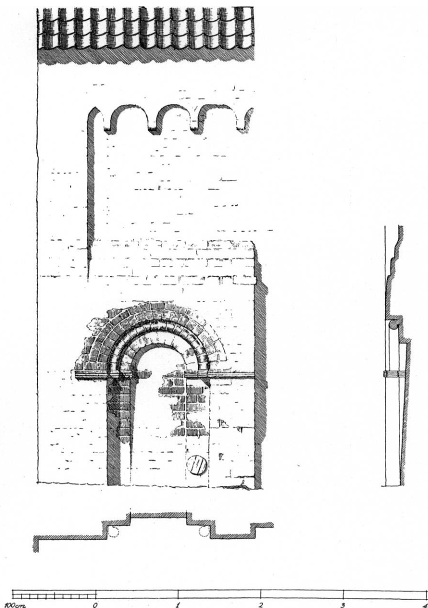
Fig. 4. Aastrup. Præstedør i Koret. 1:50. Målt af Jens Carlsen 1943.
