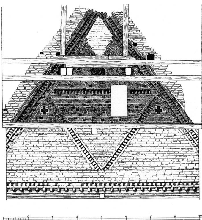
Fig. 5. Aastrup. Skibets vestgavl. 1:100. Målt af J.C.Andersen 1943.
