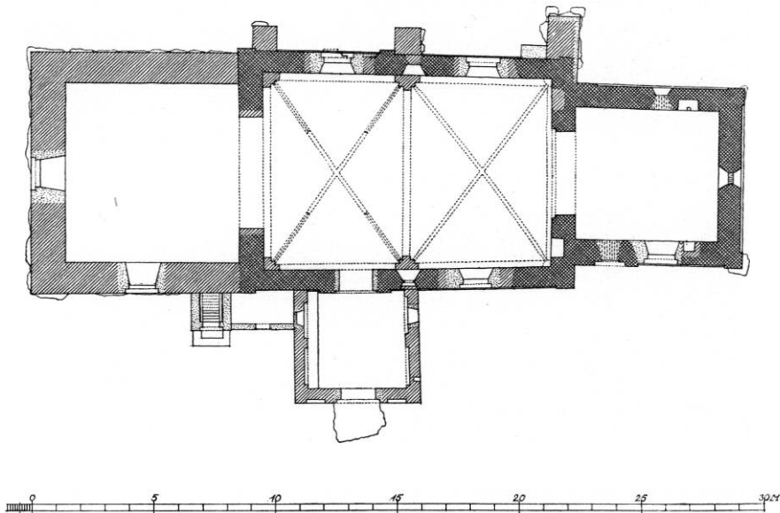
Fig. 2. Aastrup. Plan. 1:300. Målt af Jens Carlsen 1943.
