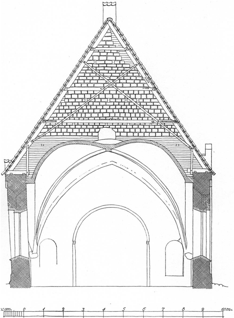
Fig. 6. Aastrup. Snit, nord-syd, gennem skibet. 1:100. Målt af Vald. Christensen 1943.
