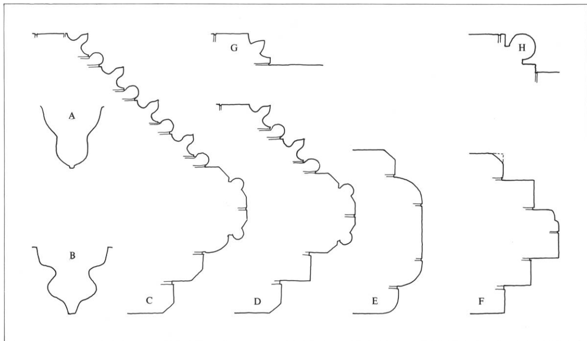
Fig. 45. Profiler. a. Ribbe i vestforlængelse, kor, skib og nordre sideskib (s. 1286, 1295, 1298 og 1303). b. Hængestav i kor (s. 1295). 1:10. c. Vindue i korets østgavl (s. 1289). d. Vindue i korets sydside (s. 1291). e. Vindue i gavlen af nordre korsarm (s. 1274). f. Nordvindue i vestforlængelsens vestre fag (s. 1270). g. Spidsbuet blænding i korets gavl (s. 1293). h. Cirkelblænding i korets gavl (s. 1293). 1:20. a-b målt af HJ 1997, c-f af Thomas Hillerup 1999 og g-h af Charles Christensen 1926. Tegnet af HJ 1999. - Mouldings a. Rib in the chancel, nave and north side aisle. b. Shaft in the chancel. c. Window in the east gable of the chancel. d. Window in the south side of the chancel. e. Window in the gable of the north transept. f. Window to the north in the west bay of the west extension. g. Pointed recess in the gable of the chancel. h. Circular recess in the gable of the chancel.
