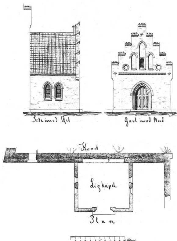
Fig. 90. Udkast til ligkapel, nu sakristi (s. 1309f.). 1:300. Påtegnet Carl Lendorff juni 1879. Rigsarkivet. - Proposal for the mortuary, now sacristy.
