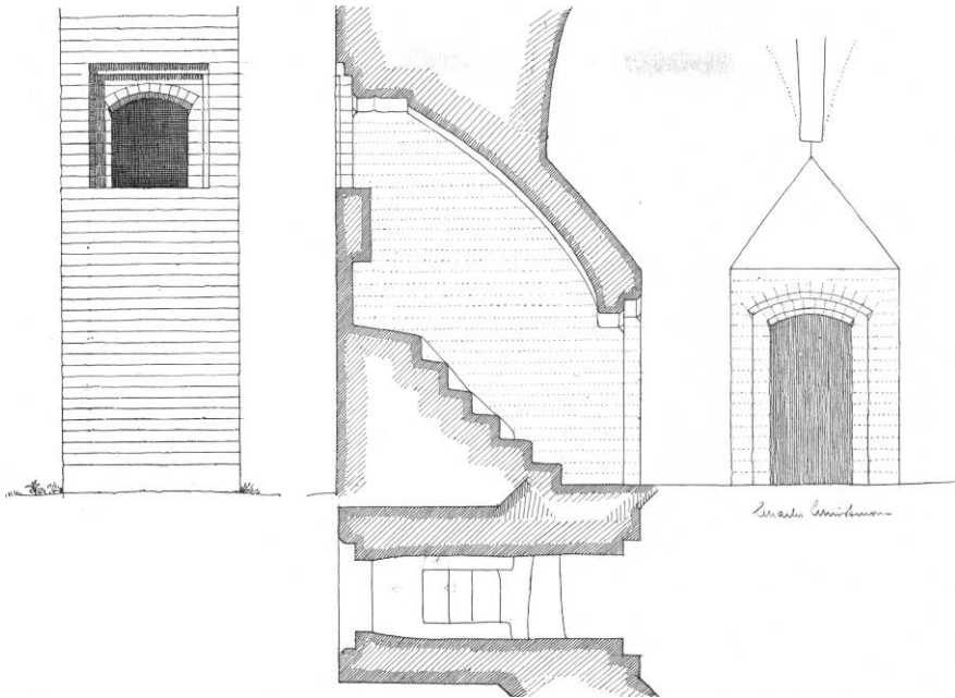
Fig. 55. Søndre sideskibs hjørnepille med udvendig prædikestol (s. 1278f.). Plan, snit og facader, jfr. fig. 104, 329. 1:75. Målt og tegnet af Charles Christensen 1926. - South side aisle's corner pillar with external pulpit, cf. figs. 104, 329.
