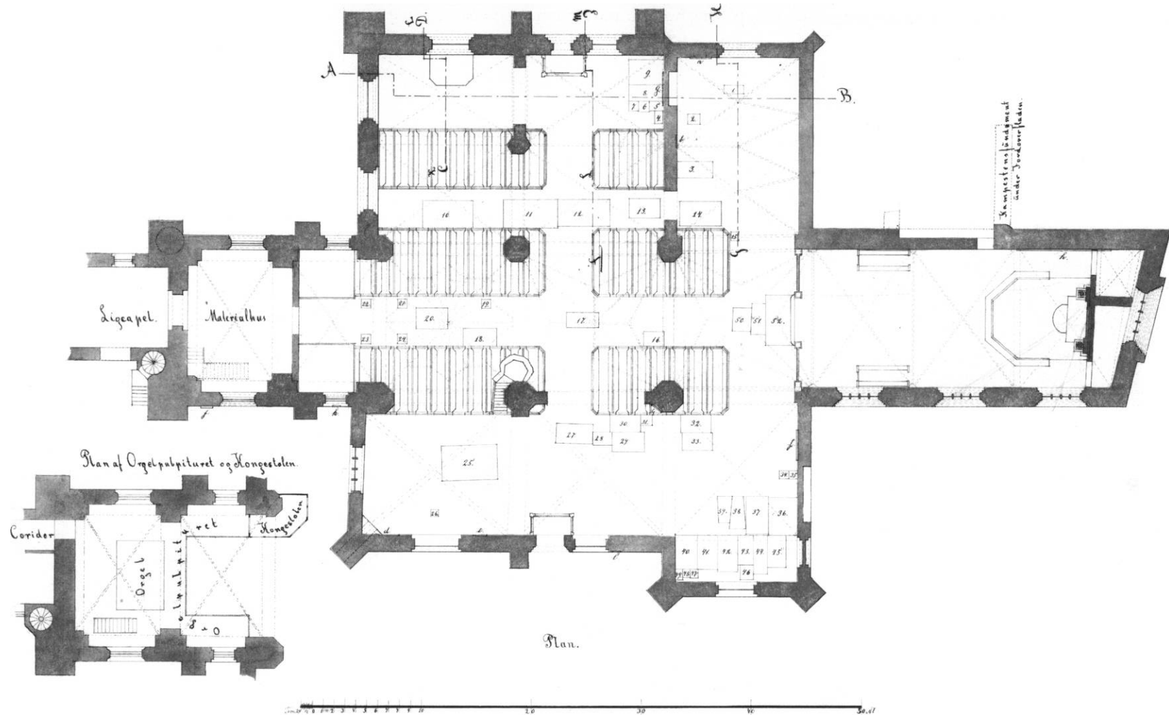
Fig. 36. Plan. 1:300. Målt og tegnet af Carl Lendorf under medvirken af L. A. Winstrup. Påtegnet febr. 1877. - Plan.
