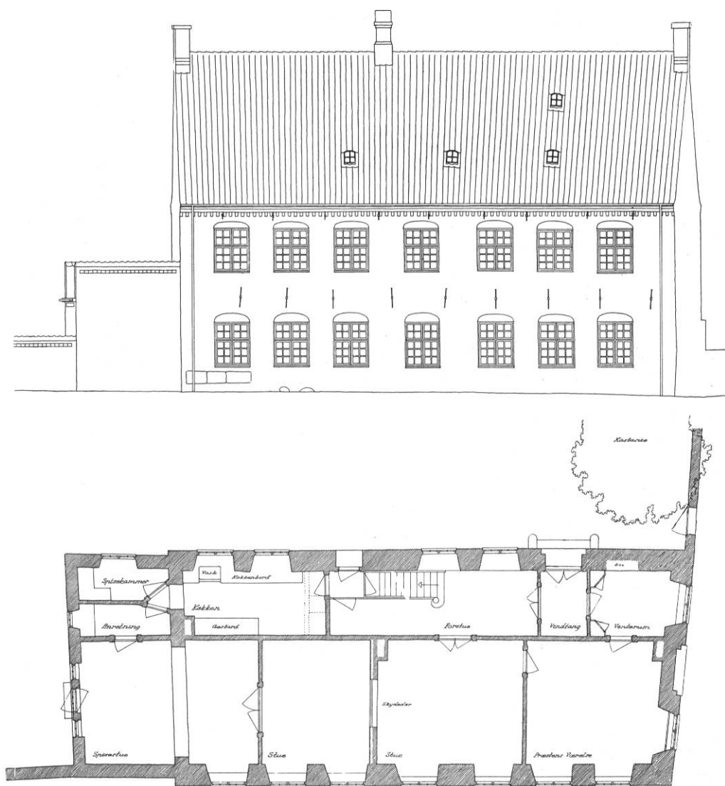
Fig. 11. S. Hans præstegård (s. 1231f., 1237f.). Plan og sydfacade. 1:200. Målt og tegnet af Jørgen Stærmose 1941. Efter Hermansen . - St. Hans' rectory. Ground-plan and south facade.
