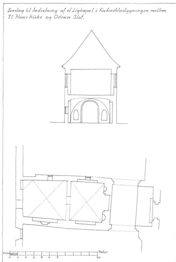
Fig. 97. Forslag til indretning af ligkapel i løngangens underetage (s. 1318). Plan og snit mod øst. 1:300. Knud Lehn Petersen o. 1945. Ebbe Lehn Petersens arkiv. - Proposal for the arrangement of the mortuary in the lower floor of the communication gallery. Plan and section to the east.
