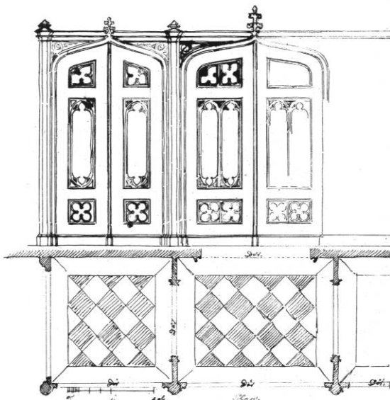
Fig. 170. Plan og opstalt af projekteret vindfang i nygotisk stil. Tegning af C. A. Møller, 1852 (s. 1389). - Plan and elevation for projected porch in neo-gothic style. Drawing by the architect C. A. Møller, 1852.
