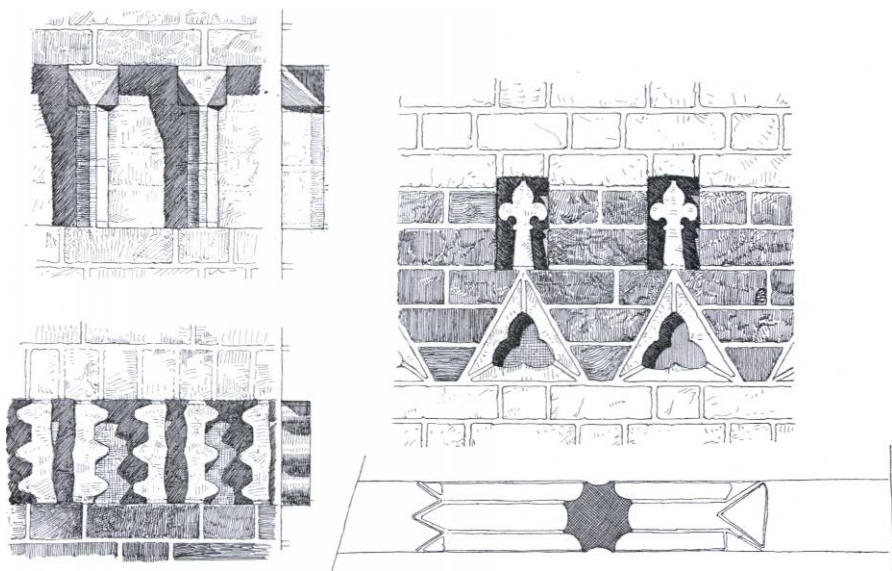
Fig. 66. Blændingsfriser på korets facader, jfr. fig. 37, 38 og 40, samt facade og snit af ankerbjælke i koret, jfr. fig. 307 (s. 1291f., 1295). 1:20. Målt og tegnet af Charles Christensen 1926. - Recessed friezes on the east and north walls of the chancel, cf. figs. 37, 38 and 40, together with facade and section of the anchored beam in the chancel, cf. fig. 307.
