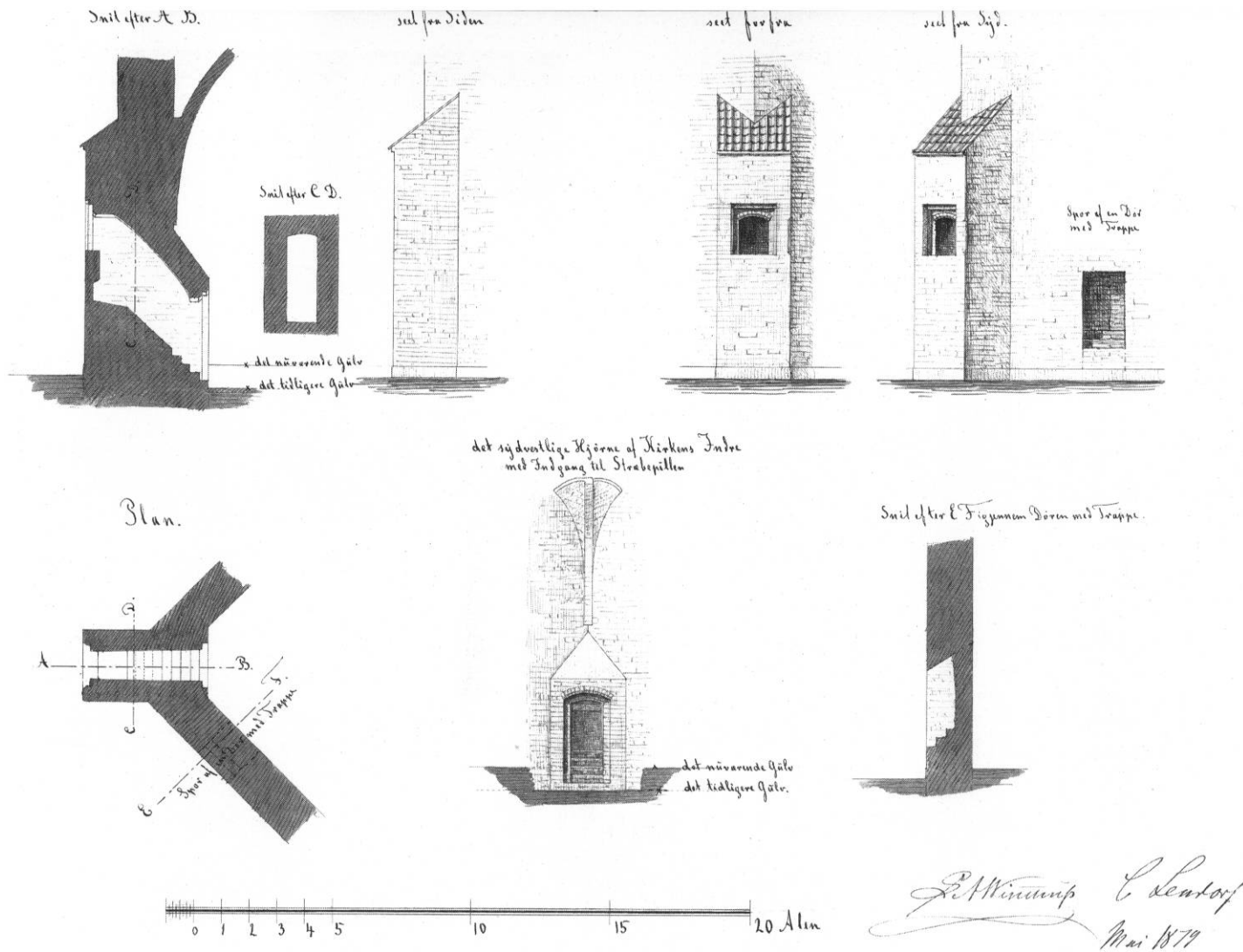
Fig. 104. Søndre sideskibs hjørnepille med udvendig prædikestol samt \dagger dør til lukket stol (s. 1278f., 1385). 1:150. Plan, snit og facader, målt og tegnet af Carl Lendorf under medvirken af L. A. Winstrup. Påtegnet maj 1879. - South side aisle's corner pillar with external pulpit and \dagger door to a pew gallery.
