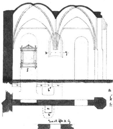
Fig. 83. Diverse snit af nordre korsarm og nordkapellet inden nedbrydningen af sidstnævntes to nordlige fag under hovedrestaurationen 1877-80. 1:300. Målt og tegnet af Carl Lendorf under medvirken af L. A. Winstrup. Påtegnet maj 1879. - Diverse sections of the north transept and north chapel before the demolition of the latter's two northernmost bays upon the restoration of 1877-80.
