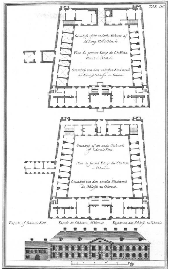
Fig. 96. Planer og havefacade af Odense Slot og løngangen til kirken. Efter Lauritz de Thurah, Den Danske Vitruvius , Kbh. 1749. - Plans and garden facade of Odense Castle and the communication gallery leading to the church. After Lauritz de Thurah, Den Danske Vitruvius , Cpgn. 1749.
