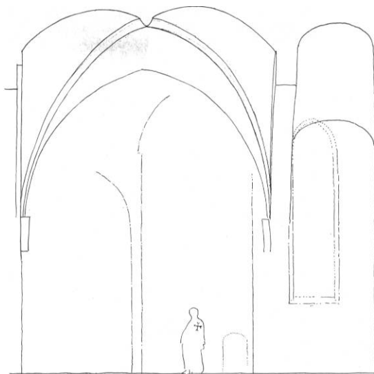
Fig. 50. Rekonstruktion af søndre korsarms østvæg med angivelse af hvælvforlæg og tilmuret, sekundært forhøjet arkadeåbning (s. 1277, 1306). 1:150. Tegnet af Charles Christensen 1926. - Reconstruction of the south transept's east wall with indication of springing points for vault, and walled up secondary, heightened arcade opening.
