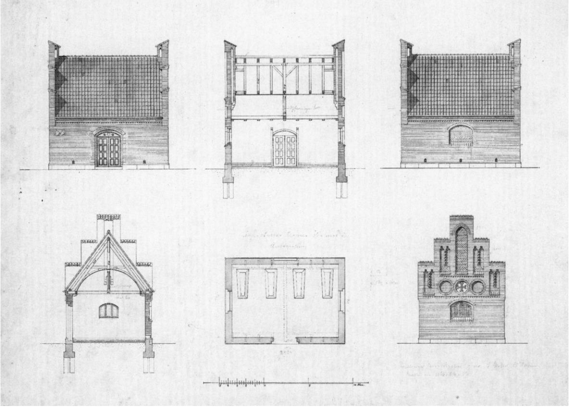
Fig. 31. †Ligekapel, opført 1906, nedrevet 1946 (s. 1253). Plan, snit og facader ved Vilh. Petersen. Ebbe Lehn Petersens arkiv. - †Mortuary, built 1906 and pulled down in 1946.
