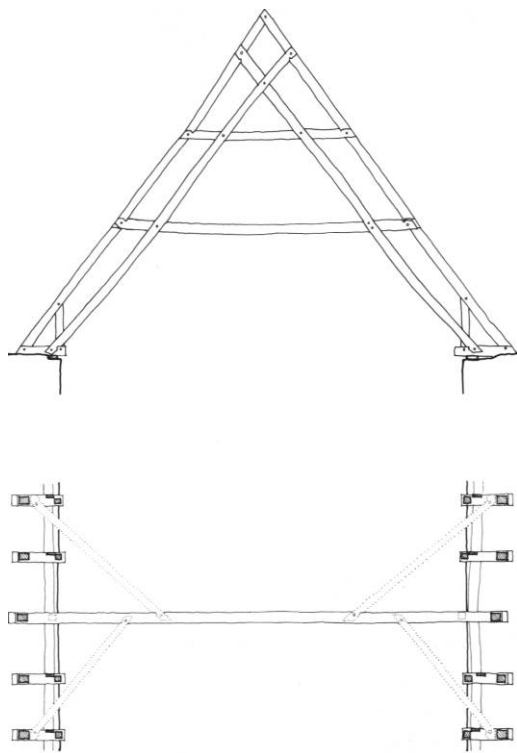
Fig. 109. Plan og opstalt af spærfag i koret mellem 2. og 3. fag. Tømmeret er ifølge dendrokronologisk datering fældet i 1460'erne (s. 1334). 1:150. Målt og tegnet af Trine Gregers og Thomas Hillerup 1998. - Plan and elevation of truss in the chancel between the second and third bays. The timber was felled in the 1460s according to dendrochronological dating analyses.
