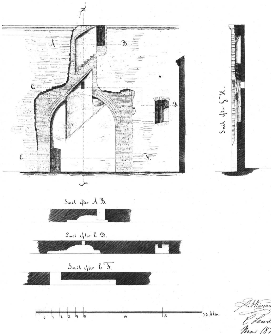
Fig. 91. Spor af tsakristi og ttrappehus ved korets nordside, fremkommet under hovedrestaurationen 1877-80 (s. 1312f., 1328). 1:150. Planer, facade og snit ved Carl Lendorf under medvirken af L.A. Winstrup. Påtegnet maj 1879. - Traces of tsacristy and tstairs annex on the north wall of the chancel, exposed during the restoration 1877-80.
