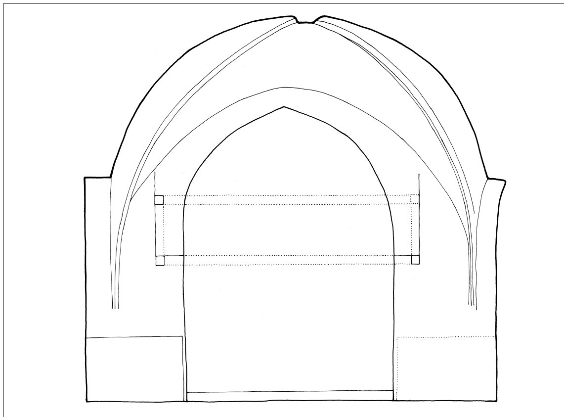
Fig. 28. Tværsnit 1:150 gennem skibet set mod øst. Triumfmuren med rekonstrueret \dagger lektorium (s. 2123 ff.). Målt af Thomas Hillerup 2009, suppleret og tegnet af Thomas Bertelsen 2009. – Cross-section through the nave looking east. Chancel arch with reconstructed \dagger gallery.
