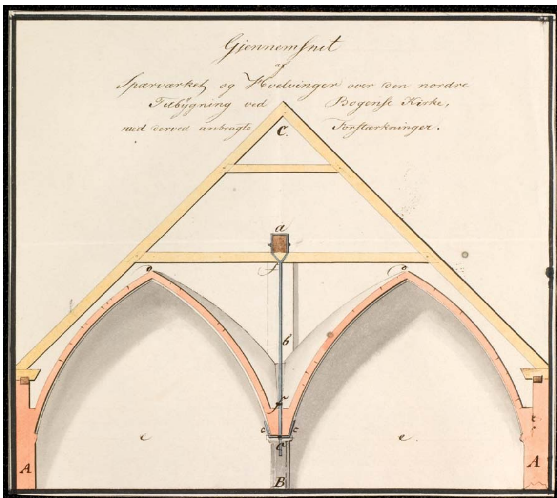
Fig. 35. Principtegning af tagkonstruktionen i nordre korsarm, med forslag til støtteanordning af tilbygningens hvelv (s. 2126). Landsarkivet for Fyn 1819. – Construction drawing of the roof structure of the north transept, with proposal for arrangement of support for the vault of the extension.
