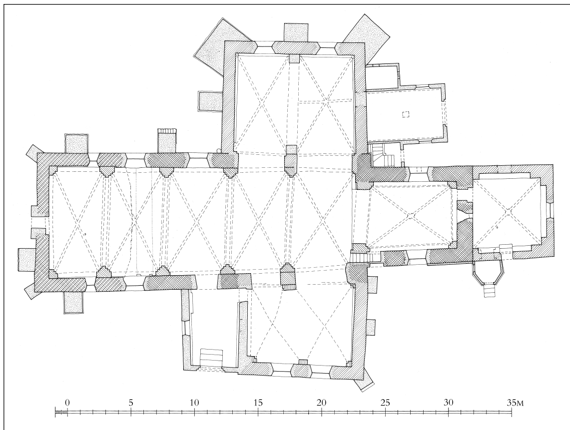
Fig. 11. Plan 1:300. Målt af Thomas Hillerup 2009, suppleret og tegnet af Thomas Bertelsen 2009. – Plan.
