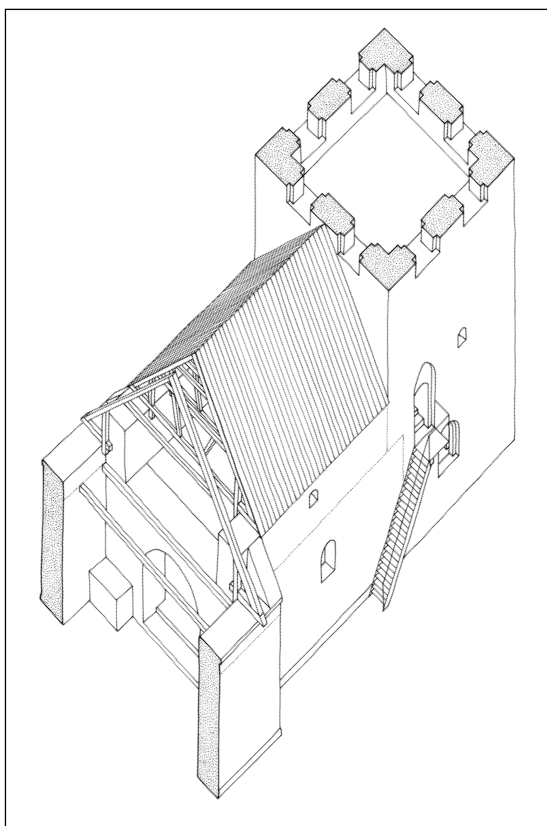
Fig. 20. Aksonometrisk principtegning af den romanske kirkes Tøvre stokværk fra o. 1455 ved sammenstødet mellem kor og skib (s. 2116 ff.). 1:300. Tegnet af Thomas Bertelsen 2009. – Axonometric drawing of the Tupper floor of the Romanesque church from c. 1455, at the junction between the chancel and the nave.
