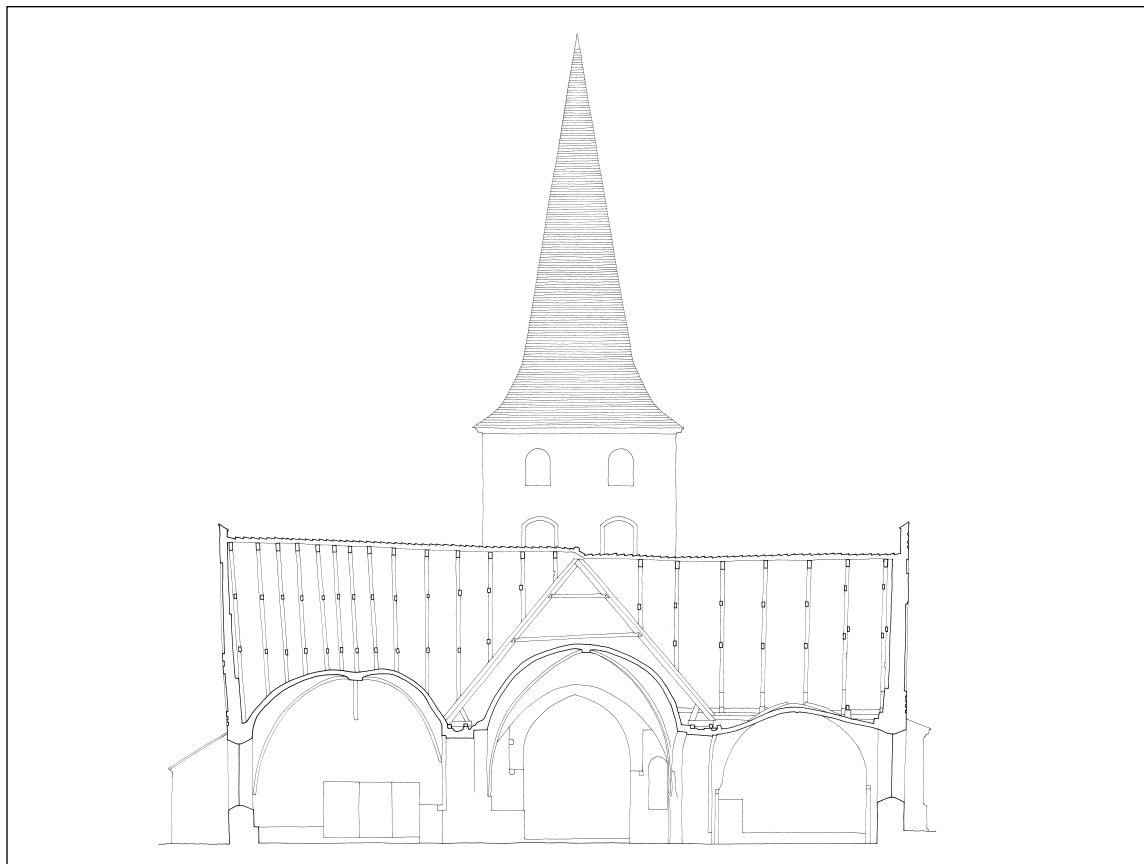
Fig. 12. Tværsnit 1:300 gennem skibet set mod øst. Målt af Thomas Hillerup 2009, suppleret og tegnet af Thomas Bertelsen 2009. – Cross-section through the nave looking east.
