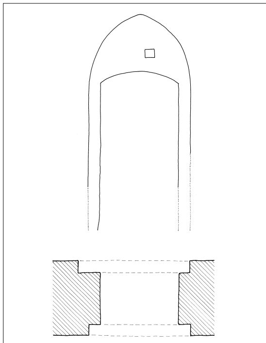
Fig. 18. Dør til mellemstokværk i tårnets sydmur (s. 2114 ff.). 1:50. Plan og opstalt af ydersiden målt og tegnet af Thomas Bertelsen 2009. – Door in the south wall of the tower, leading to the middle storey.
