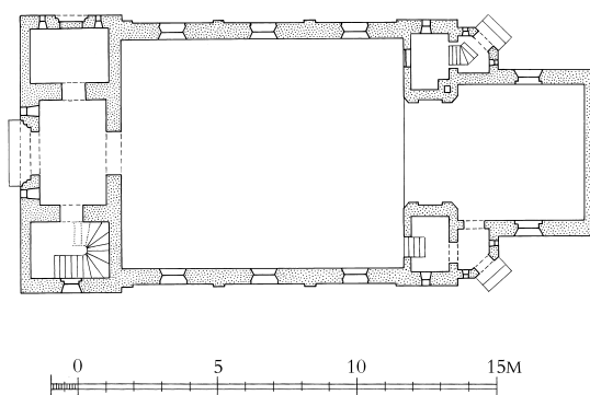
Fig. 2. Plan. 1:300. Målt af H. P. Knudsen, suppleret og tegnet af Merete Rude 2014. – Ground plan.
