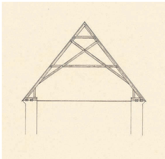
Fig. 14. Spærfag i skibets tagværk (s. 4278). 1:150. Målt og tegnet af Erik Schiødt 1884. – Scale drawing of truss in the roofing of the nave.
