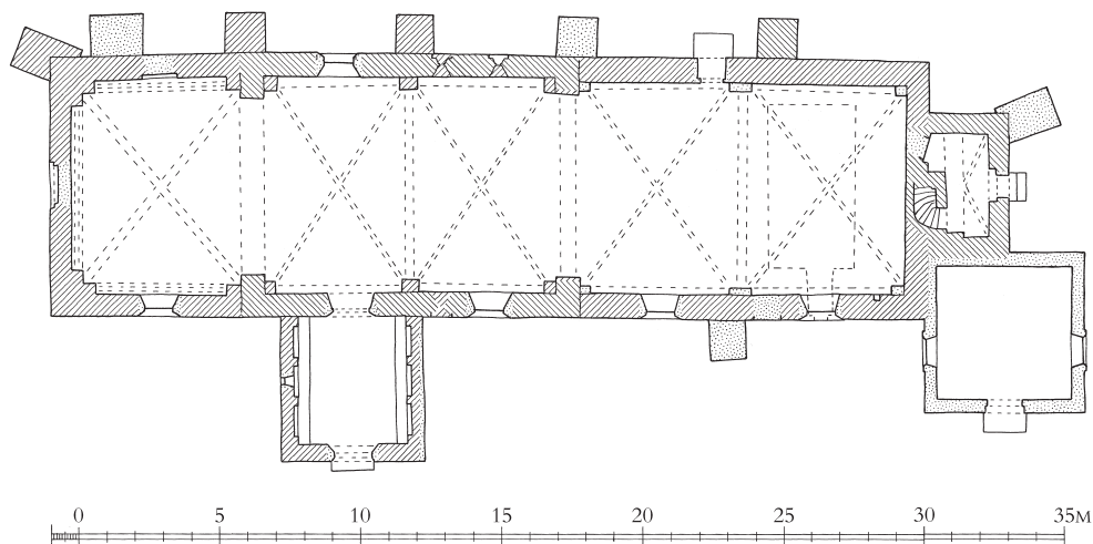
Fig. 5. Plan. 1:300. Målt af Lehn Petersens Tegnesteue 1967, suppleret af Kirstin Eliassen og tegnet af Freerk Oldenburger 2018. Signaturforklaring s. 11. – Plan. Key on p. 11.
