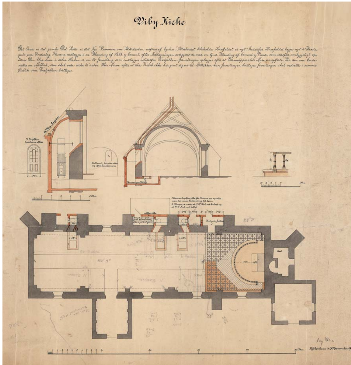
Fig. 65. Projekt til nyt varmeanlæg (s. 4545) ved arkitekt Aug. Klein 1891. 1:300. I NM. – Project for new heating system by the architect Aug. Klein.
