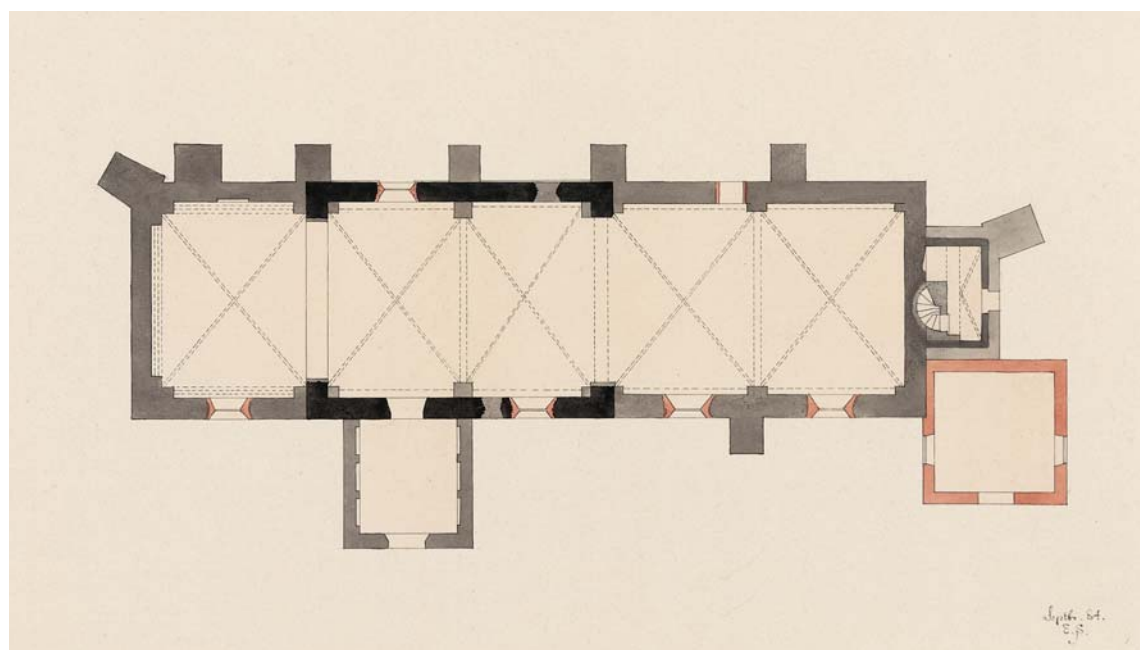
Fig. 27. Plan. 1:300. Målt og tegnet af Erik Schiødte 1884. – Plan.
