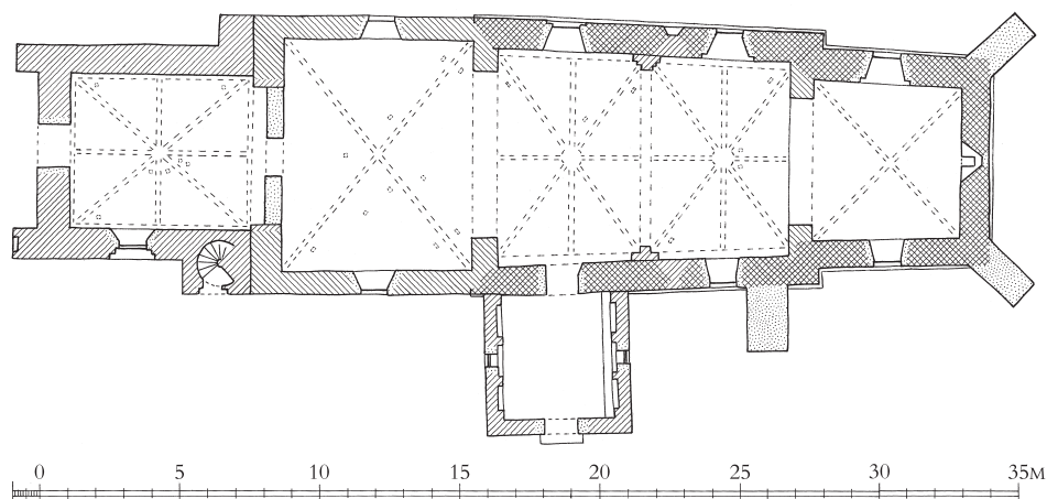
Fig. 5. Plan. 1:300. Målt af Lehn Petersens Tegnestue 1995, suppleret af Kirstin Eliassen og tegnet af Freerk Oldenburger 2018. Signaturforklaring s. 11. – Plan. Key on p. 11.
