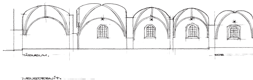
Fig. 10. Længdesnit set mod nord. 1:300. Målt og tegnet af Lehn Petersens Tegnestue o. 1995. – Longitudinal section looking north.
