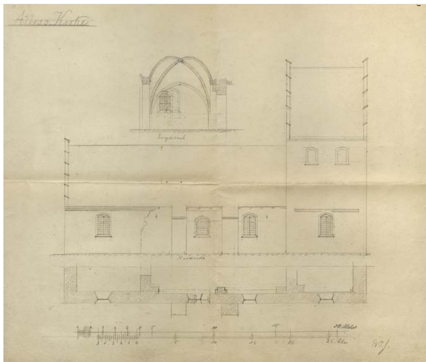
Fig. 12. Længdesnit i skibets 1. fag set mod nord, opstalt af kirkens nordfacade samt udsnit af plan. 1:300. Målt og tegnet af N. P. Jensen o. 1912. I Historiens Hus, Odense. – Longitudinal section of nave, 1. bay, looking north, elevation of north facade and plan.
