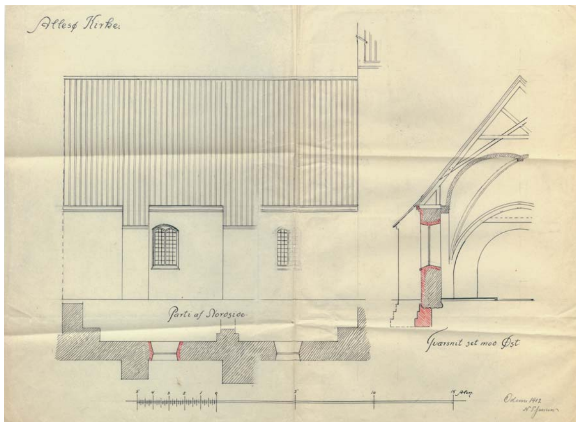
Fig. 13. Detaljer af skibets nordside. Opstalt af nordfacade, udsnit af plan samt nordre halvdel af tværsnit set mod øst. 1:150. Målt og tegnet af N. P. Jensen 1912. I Historiens Hus, Odense. – Details of nave, north side. Elevation of north facade, plan and northern half of cross-section looking east.
