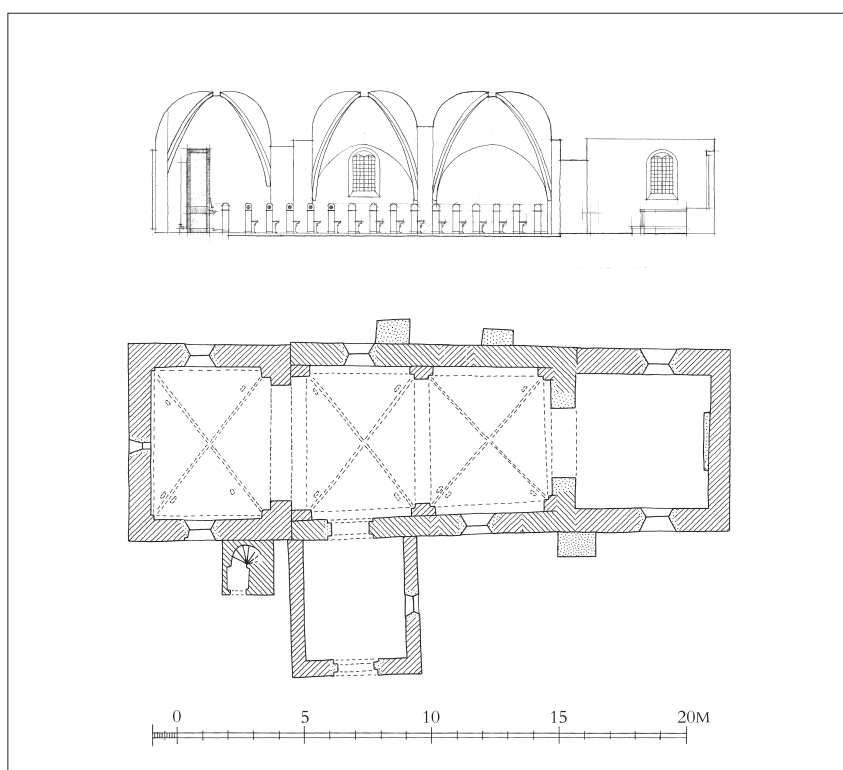
Fig. 4-5. 4. Længdesnit set mod nord. 1:300. Målt og tegnet af Lehn Petersens Tegnestue 1983. I NM. 5. Plan. 1:300. Målt af Kirstin S. Eliassen 2019 med udgangspunkt i tegning ved Lehn Petersens Tegnestue 1983, tegnet af Freerk Oldenburger 2019. Signaturforklaring s. 11. — 4. Longitudinal section looking north. 5. Plan. Key on p. 11.
