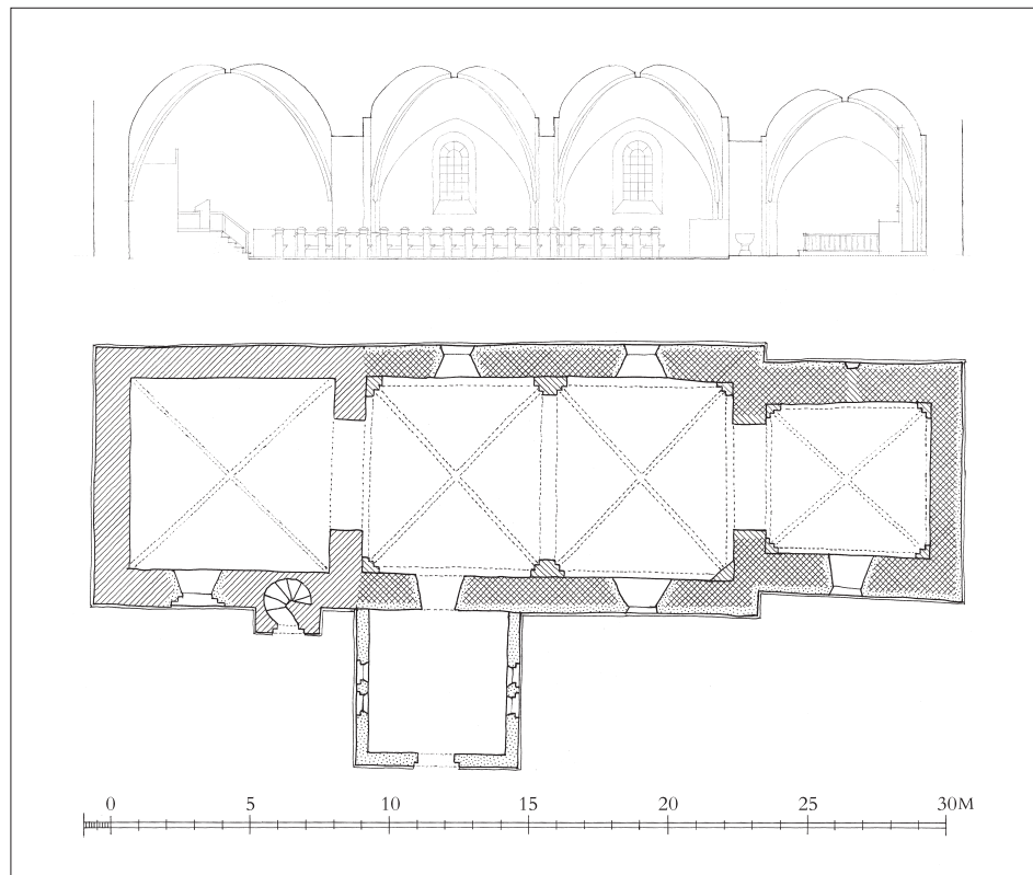
Fig. 7-8. 7. Længdesnit set mod nord. 1:300. Målt og tegnet af Lehn Petersens Tegnestue 1988. 8. Plan. 1:300. Målt af Lehn Petersens Tegnestue 1988 og tegnet af Martin Wangsgaard Jürgensen 2019. Signaturforklaring s. 11. – 7. Longitudinal section looking north. 8. Plan. Key on p. 11.
