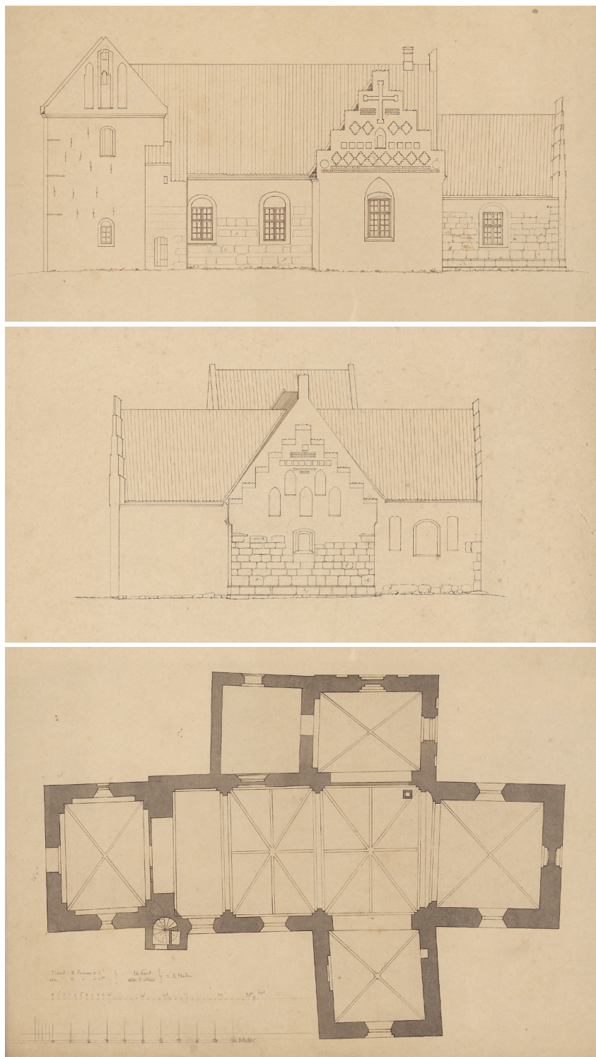
Fig. 8a-c. Opstalter af syd- og østfacade samt plan. 1:300. Målt og tegnet af J. Vilh. Petersen eller Alfred Petersen 1888. I NM. – Elevations of south and east facades and plan.
