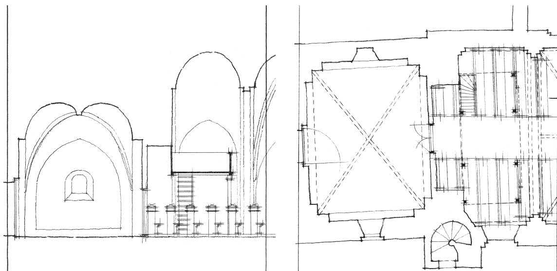
Fig. 58-59. †Orgelpulpitur, 1917. 1:150. Målt og tegnet af Knud, Erik og Ebbe Lehn Petersen Arkitekter 1963. 58. Snit set mod nord. 59. Plan. – † Organ gallery , 1917. 58 Section looking north. 59. Plan.
