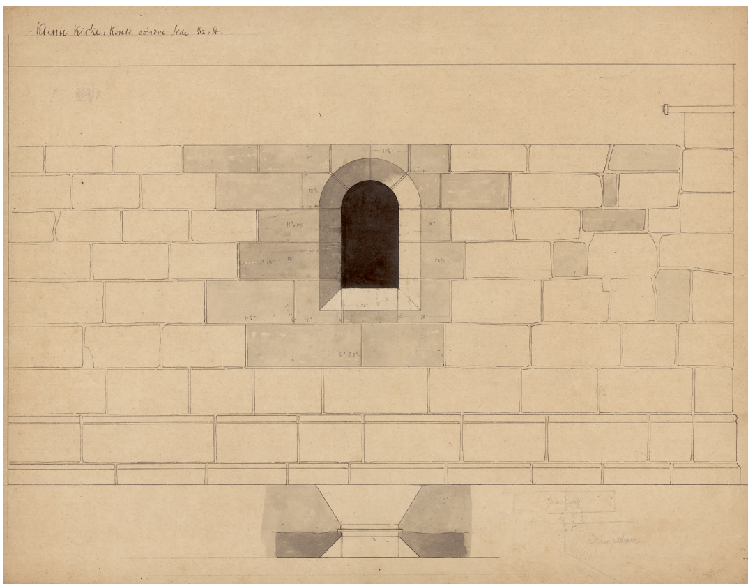
Fig. 32. Forslag til nyt vindue i korets sydside (s. 5530). 1:50. Tegnet af J. Villh. Petersen 1888. I NM. – Proposal for new window in the south facade of the chancel.
