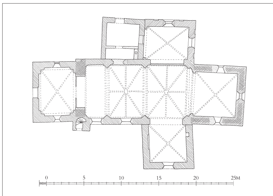
Fig. 7. Plan. 1:300. Målt af J. Vilh. Petersen eller Alfred Petersen 1888 (jf. fig. 8c), suppleret af Kirstin Eliassen 2019 og tegnet af Freerk Oldenburger 2020. Signaturforklaring s. 11. – Plan. Key on p. 11.
