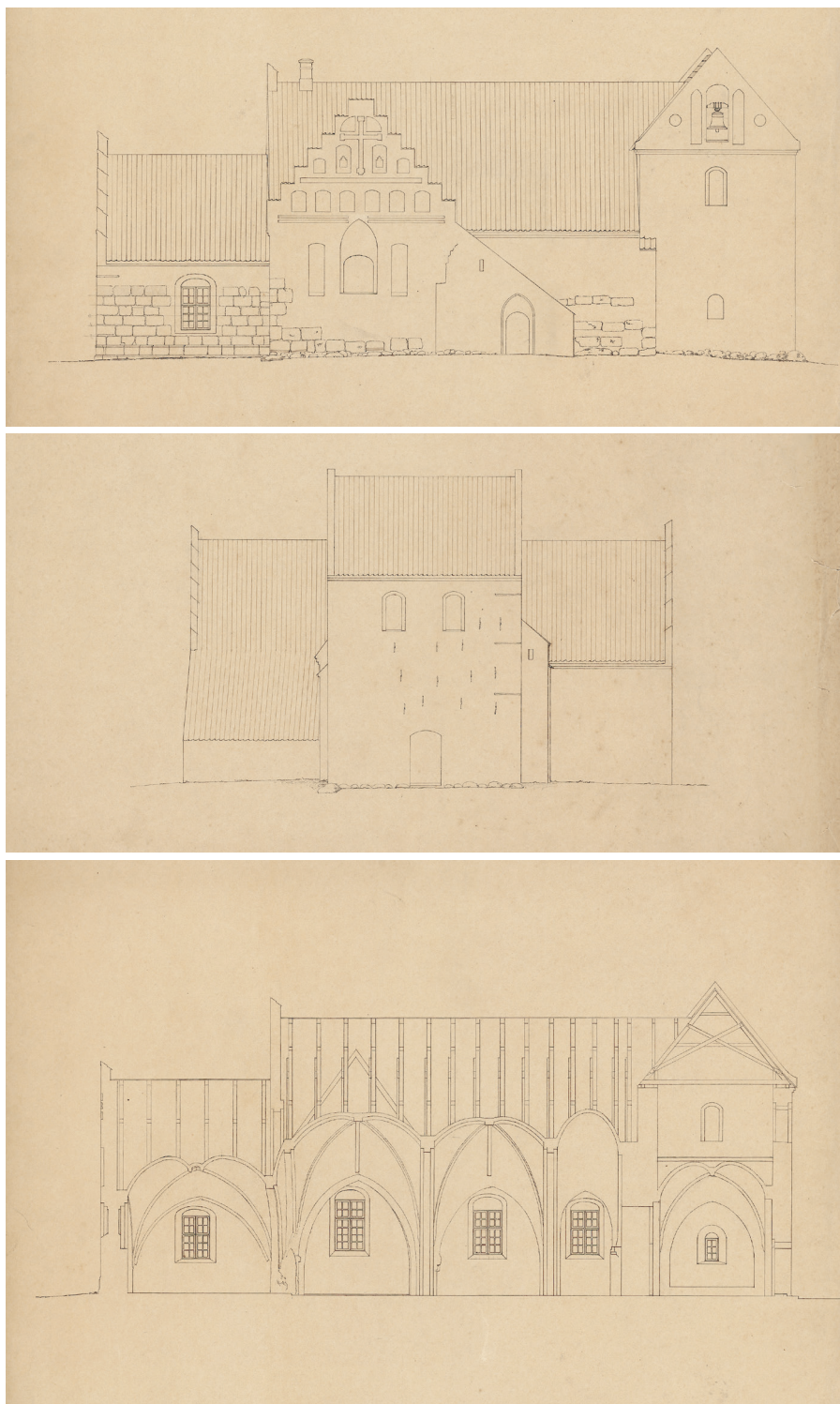
Fig. 8d-f. Opstalter af nord- og vestfacade samt længdesnit set mod syd. 1:300. Målt og tegnet af J. Vilh. Petersen eller Alfred Petersen 1888. I NM. — Elevations of north and west facades and longitudinal section looking south.
