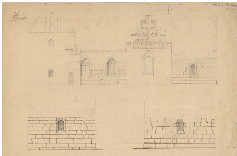
Fig. 31. Opstalt af sydfacade med forslag til nye vinduer (s. 5530). 1:300. Opstalter af korets syd- og nordfacader med forslag til nye vinduer. Ca. 1:190. Tegnet af J. Vilh. Petersen 1888. I NM. – Elevation of south facade with proposal for new windows and elevations of south and north facades of the chancel with proposal for new windows.
