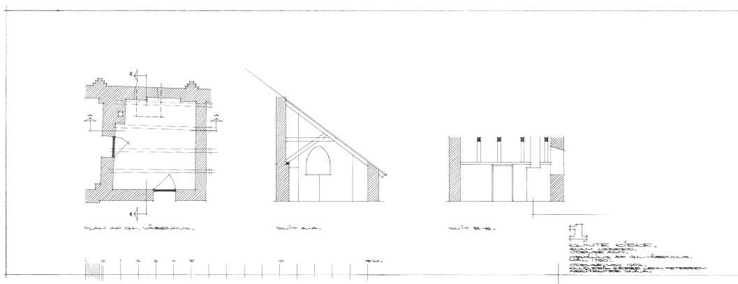
Fig. 69a-c. Opmålinger af våbenhuset (s. 5520). 1:300. Knud, Erik og Ebbe Lehn Petersen arkitekter 1962. I NM. a. Plan. b. Snit set mod syd. c. Snit set mod øst. – Scale drawings of porch. a. Plan. b. Section looking south. c. Section looking east.
