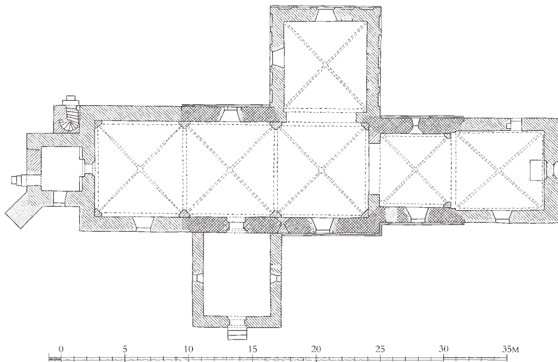
Fig. 6. Plan. 1:300. Målt af Lehn Petersens Tegnestue u.å. korrigeret og suppleret af Kirstin Eliassen og tegnet af Freerk Oldenburger 2021. Signaturforklaring s. 11. – Plan. Key on p. 11.
