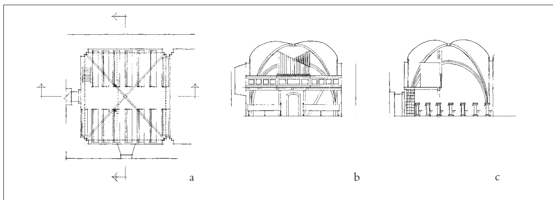
Fig. 105a-c. Opmåling af skibets vestforlængelse (s. 6006) med torgel (s. 6058), 1903. 1:300. a. Plan. b. Tværsnit set mod vest. c. Længdesnit set mod nord. Målt af Lehn Petersens Tegnestue 1970. — Scale drawing of the western extension of the nave with torgel, 1903. a. Plan. b. Cross section looking west. c. Longitudinal section looking north.
