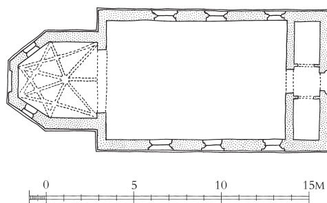
Fig. 4. Plan. 1:300. Målt af David Burmeister og Martin Wangsgaard Jürgensen, tegnet af sidstnævnte 2021. Signaturforklaring s. 11. – Plan. Key on p. 11.
