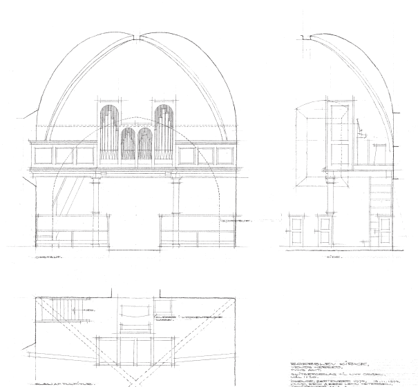
Fig. 100. Opmåling af kirkens vestende med torgel nr. 2 (s. 6699). 1:150. Tværsnit set mod vest, længdesnit set mod syd og plan. Målt og tegnet af Knud, Erik og Ebbe Lehn Petersen 1974. I NM. – Scale drawing of the west end of the church with torgel no. 2. Cross-section looking west, longitudinal section looking south, and plan.
