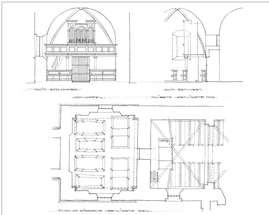
Fig. 69. Opmåling af kirkens vestende med \dagger orgel nr. 1 (s. 6699). 1:150. Tværnsnit set mod vest, længdesnit set mod syd og plan. Målt og tegnet af Knud, Erik og Ebbe Lehn Petersen 1974. I NM. – Scale drawing of the west end of the church with \dagger organ no. 1. Cross-section looking west, longitudinal section looking south, and plan.
