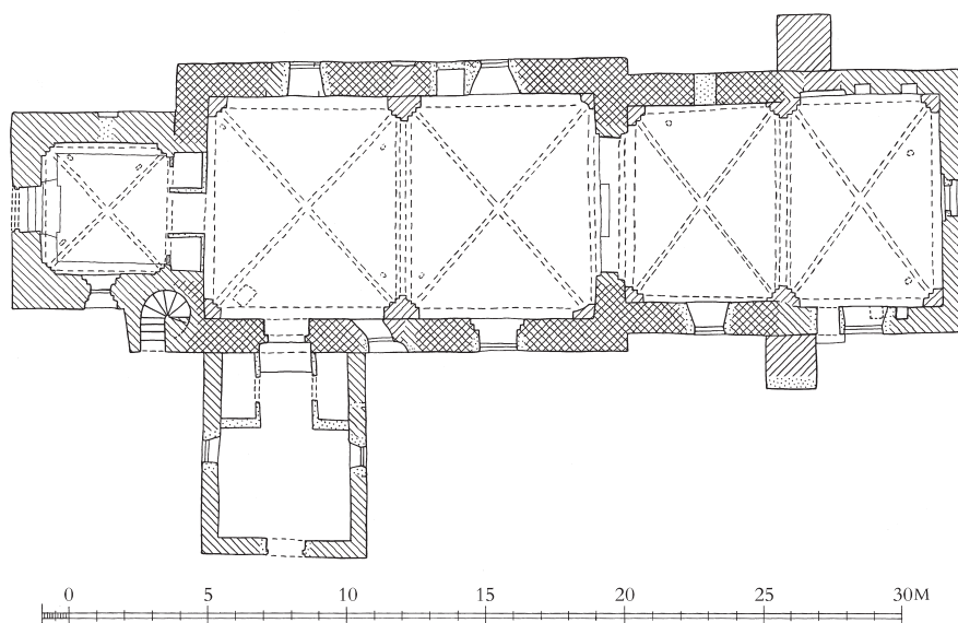
Fig. 7. Plan. 1:300. Målt af Vilhelmsen, Marxen og Bech-Jensen 1996, suppleret af Kirstin S. Eliassen og tegnet af Freerk Oldenburger 2025. Signaturforklaring s. 11 – Plan. Key on p. 11.
