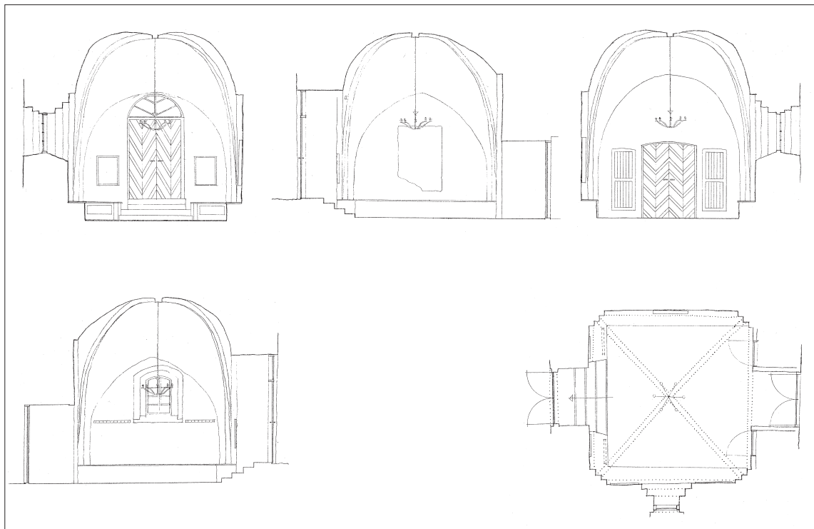
Fig. 112a-e. Forslag til restaurering af tårnrum 1997-98. 1:150. a-d. Snit set mod vest, nord, øst og syd. e. Plan. Målt og tegnet af Vilhelmsen, Marxen og Bech-Jensen 1996. – Proposal for restoration of the lower floor of the tower 1997-98. a-d. Sections looking west, north, east, and south. e. Plan.
