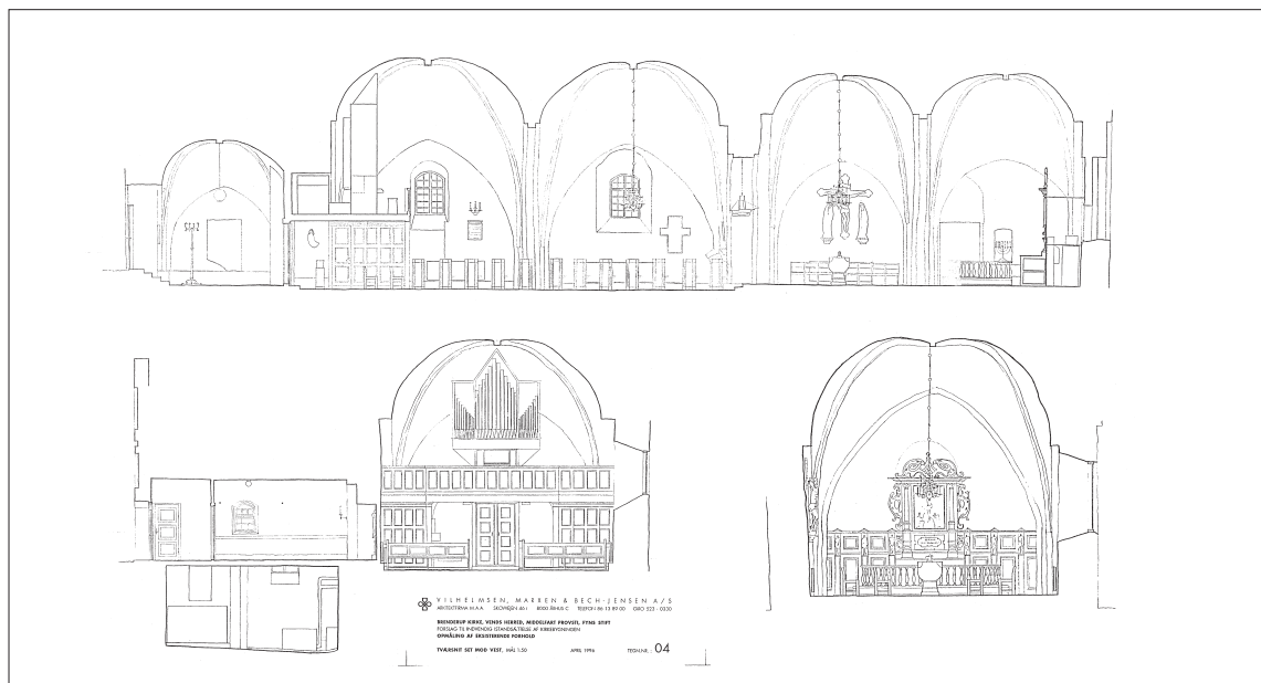
Fig. 111a-c. Opmålinger af kirken før restaureringen 1997-98. 1:300. a. Længdesnit set mod nord. b. Tværsnit af skib og våbenhus set mod vest. c. Tværsnit af kor set mod øst. Målt og tegnet af Vilhelmsen, Marxen og Bech-Jensen 1996. – Scale drawings prior to restoration 1997-98. a. Longitudinal section looking north. b. Cross-section of nave and porch looking west. c. Cross-section of chancel looking east.
