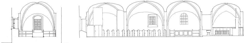
Fig. 10a-b. Opmålinger. a. Tværsnit af vestforlængelsen set mod vest. b. Længdesnit set mod nord. Målt og tegnet af Knud, Erik og Ebbe Lehn Petersen 1962 og u.å. – Scale drawings. a. Cross-section looking west. b. Longitudinal section looking north.
