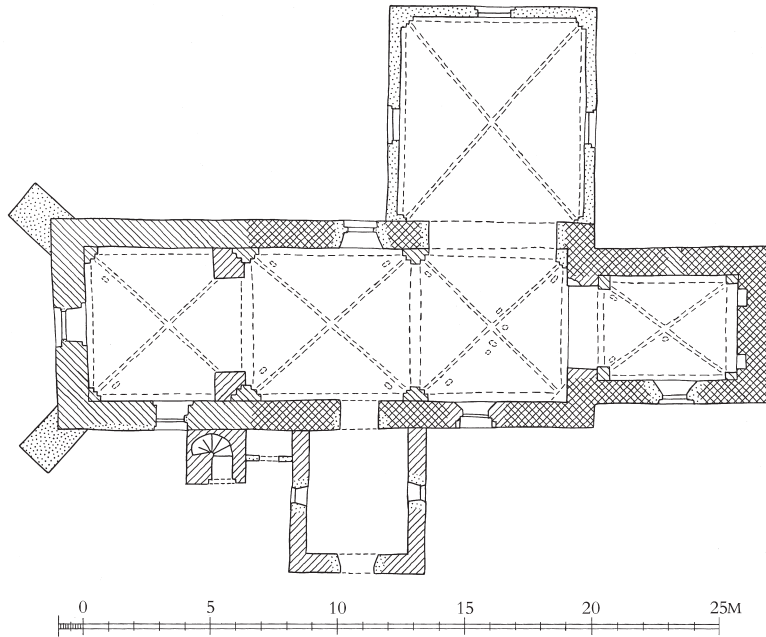
Fig. 9. Plan 1:300. Knud, Erik & Ebbe Lehn Petersen 1969. Suppleret af Kirstin S. Eliassen og tegnet af Freerk Oldenburger 2025. Signaturforklaring s. 11 – Plan. Key on p. 11.
