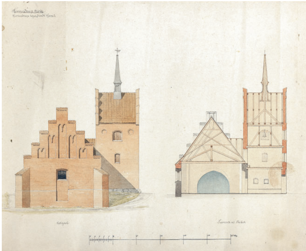
Fig. 77c–d. Ikke realiseret forslag til ombygning. 1:300. c. Opstalt af vestfacade. d. Tværsnit af skib og tårn set mod øst. Tegnet af J. Vilh. Petersen o. 1892. I Humlemagasinet, Harndrup. – Sketch for unrealized rebuilding. c. Elevation of west facade. d. Cross-section through the nave and tower looking east.
