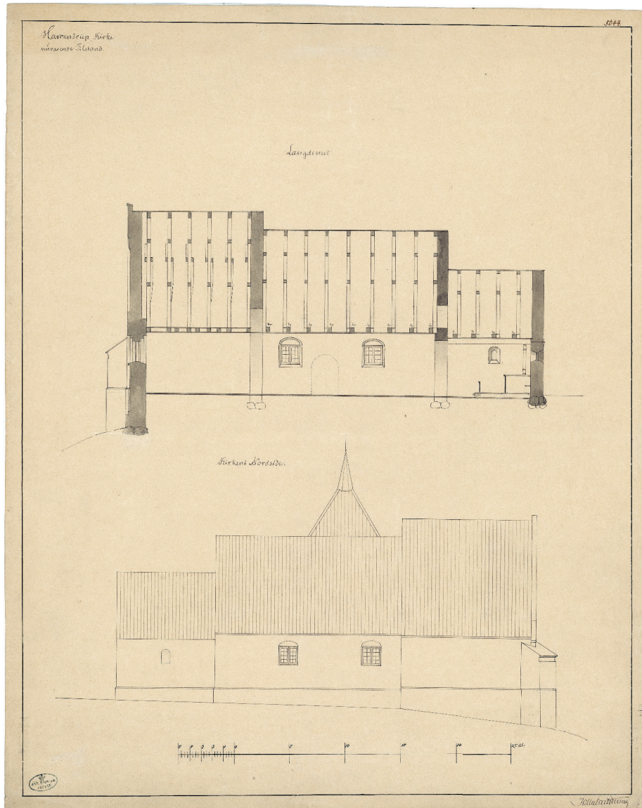
Fig. 24c-d. Opmålinger af kirken o. 1885-92. 1:300. c. Længdesnit set mod nord. d. Opstalt af nordfacaden. Målt og tegnet af J. Vilh. Petersen. I NM – Scale drawings of the church c. 1885-92. c. Longitudinal section looking north. d. Elevation of the north facade.
