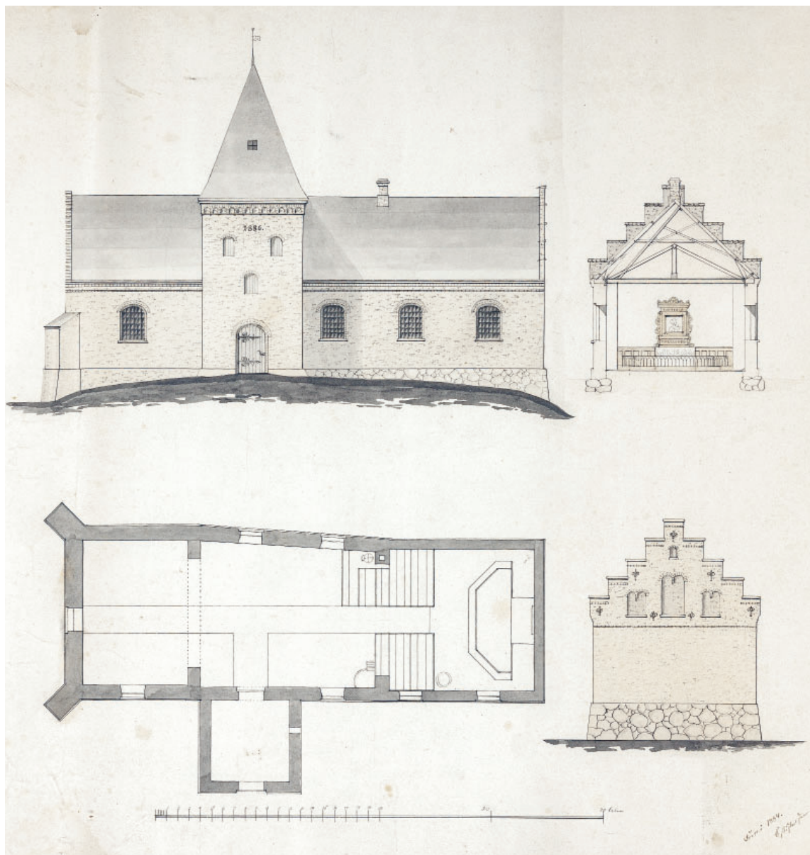
Fig. 75a-d. Forslag til ombygning. 1:300. a. Opstalt af sydfacaden. b. Tværsnit set mod øst. c. Plan. d. Opstalt af østfacaden. Tegnet af C. Michelsen 1884. I Humlemagasinet, Harndrup. – Proposal for rebuilding. a. Elevation of the south facade. b. Cross-section looking east. c. Plan. d. Elevation of the east facade.
