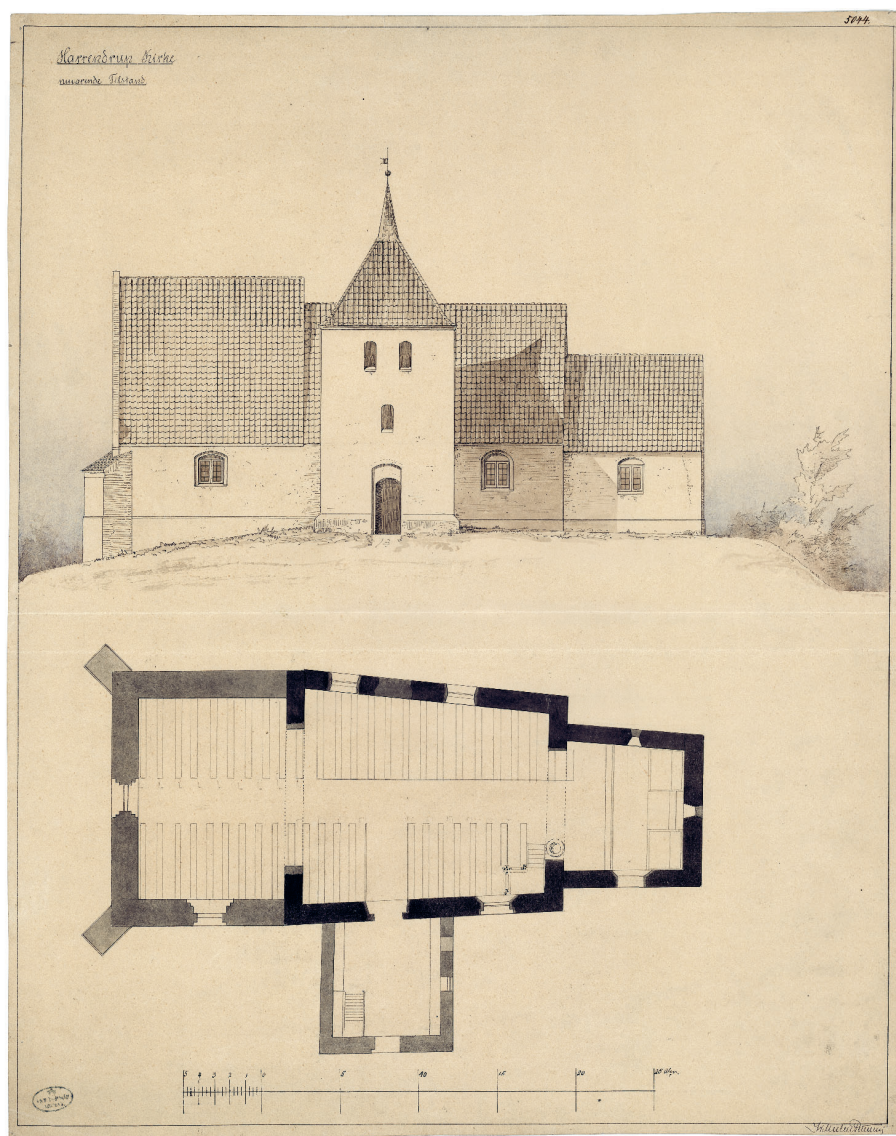
Fig. 24a-b. Opmålinger af kirken o. 1885-92. 1:300. a. Opstalt af sydfacaden. b. Plan. Målt og tegnet af J. Vilh. Petersen. I NM – Scale drawings of the church c. 1885-92. a. Elevation of the south facade. b. Plan.
