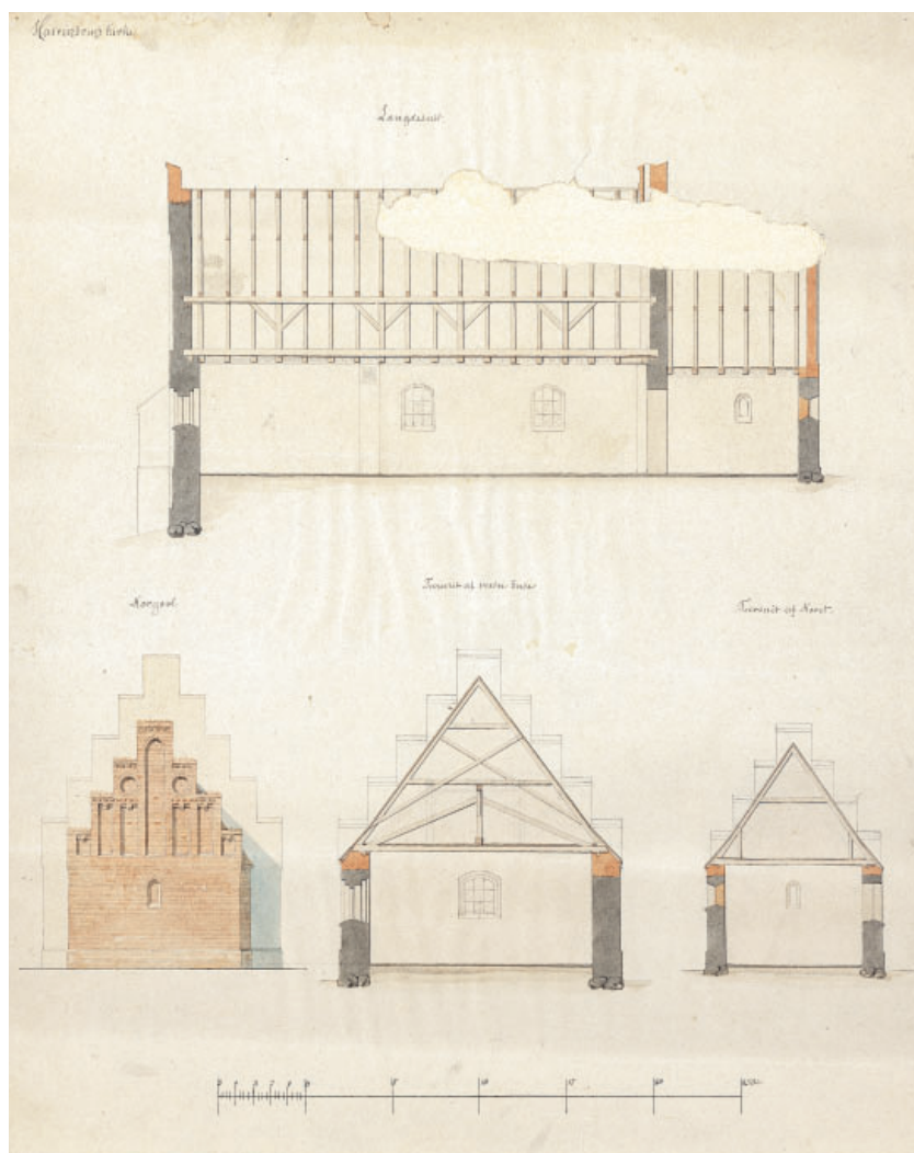
Fig. 77e-h. Ikke realiseret forslag til ombygning. 1:300. e. Længdesnit set mod nord. f. Opstalt af østfacade. g. Tværsnit af vestforlængelse set mod vest. h. Tværsnit af kor set mod øst. Tegnet af J. Vilh. Petersen o. 1892. I Humlemagasinet, Harndrup. – Sketch for unrealized rebuilding. e. Longitudinal section looking north. f. Elevation of east facade. g. Cross-section of western extension looking west. h. Cross-section of chancel looking east.
