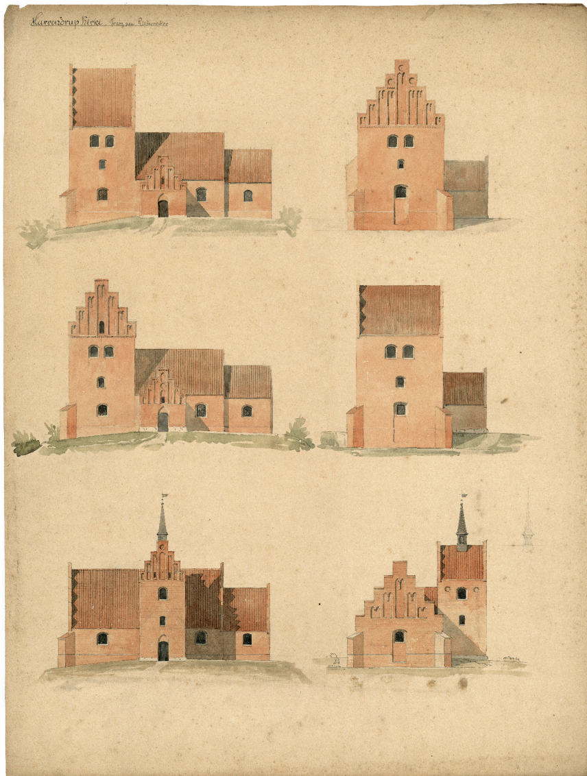
Fig. 76a-c. Skitser til urealiserede historicistiske ombygninger. a. Nygotisk tårn over vestenden og ombygning af det nuværende til et lavt, nygotisk våbenhus. b. Samme med et tværstillet vesttårn. c. Tårnet over våbenhuset opført i en højere, nygotisk skikkelse med blændingsgavl og spir. 1:600. Tegnet af J. Vilhelm Petersen o. 1892. I NM. – Sketches for unrealized historicist rebuildings. a. Neo-Gothic tower above the west end and rebuilding of the current tower to a shorter, neo-Gothic porch. b. The same, with the tower to the west rotated. c. The tower above the porch with a taller neo-Gothic appearance and a recessed gable and spire.
