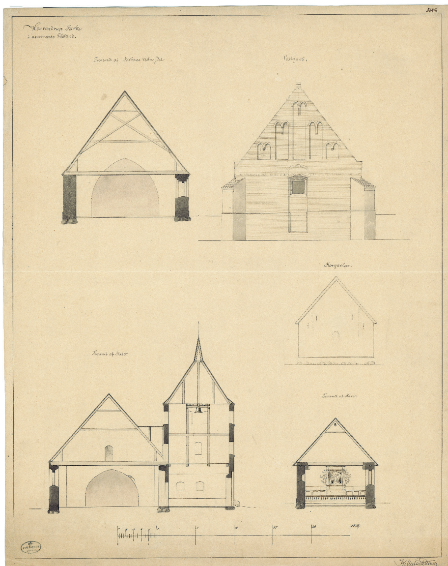
Fig. 24e-i. Opmålinger af kirken o. 1885-92. 1:300. e. Tværsnit af vestforlængelse set mod øst. f. Opstalt af vestfacaden. g. Opstalt af østfacaden. h. Tværsnit af skibet set mod øst. i. Tværsnit af koret set mod øst. Målt og tegnet af J. Vilh. Petersen. I NM – Scale drawings of the church c. 1885-92. e. Cross-section of the western extension looking east. f. Elevation of the west facade. g. Elevation of the east facade. h. Cross-section of the nave looking east. i. Cross-section of the chancel looking east.
