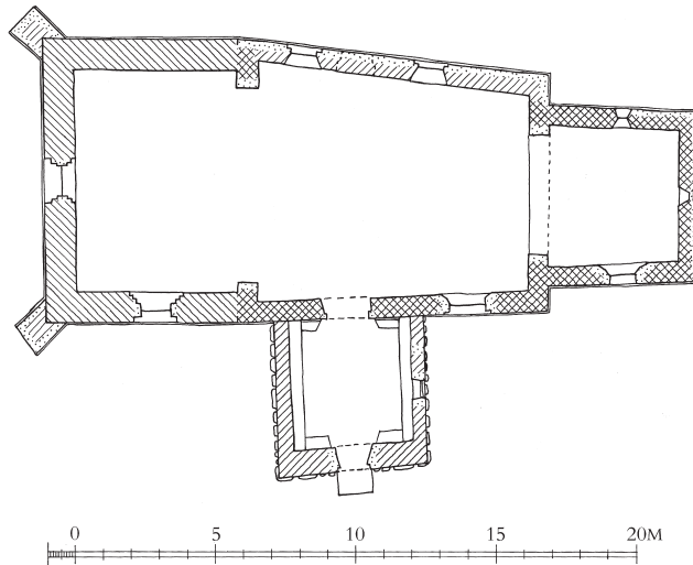
Fig. 8. Plan. 1:300. Målt og tegnet af Thomas Fjelstrup Nielsen 2024. Signaturforklaring s. 11. – Plan.
