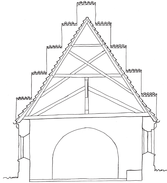
Fig. 9. Tværsnit. 1:150. Målt og tegnet af Thomas Fjelstrup Nielsen 2024. – Cross-section.
