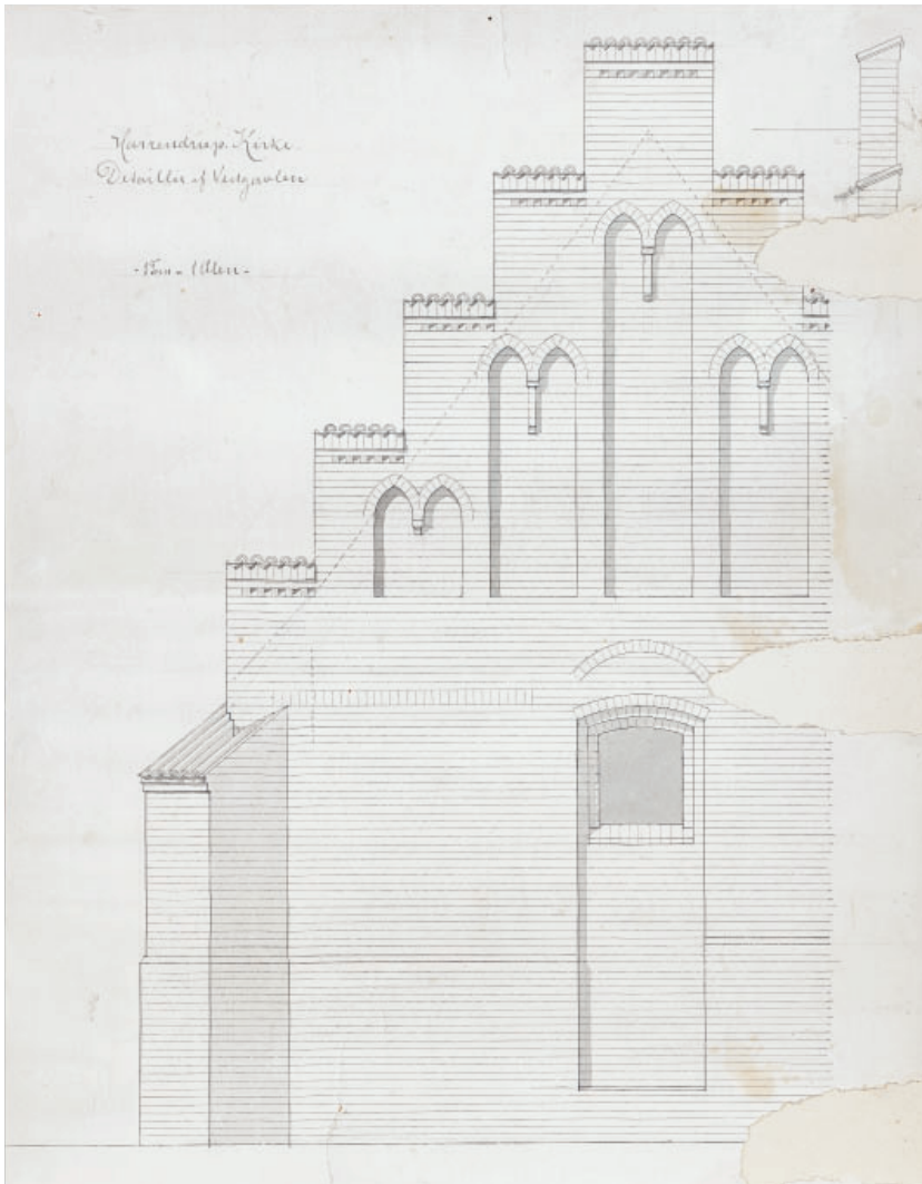
Fig. 25. Forslag til restaurering af vestforlængelsens gavl. 1:100. Tegnet af J. Vilh. Petersen o. 1892. I Humlemagasinet, Harndrup. – Proposal for restoration of the gable wall of the western extension.
