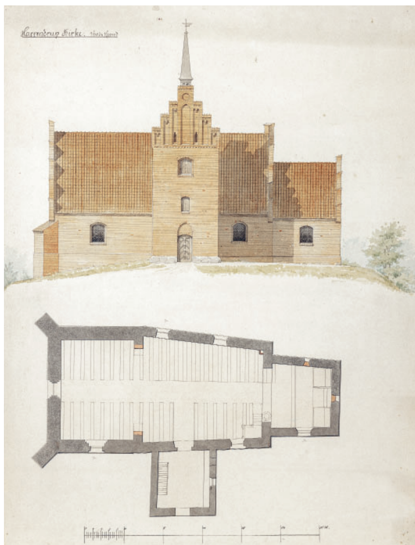
Fig. 77a-b. Ikke realiseret forslag til ombygning. 1:300. a. Opstalt af sydfacade. b. Plan. Tegnet af J.Vilh. Petersen o. 1892. I Humlemagasinet, Harndrup. – Sketch for unrealized rebuilding. a. Elevation of south facade. b. Plan.
