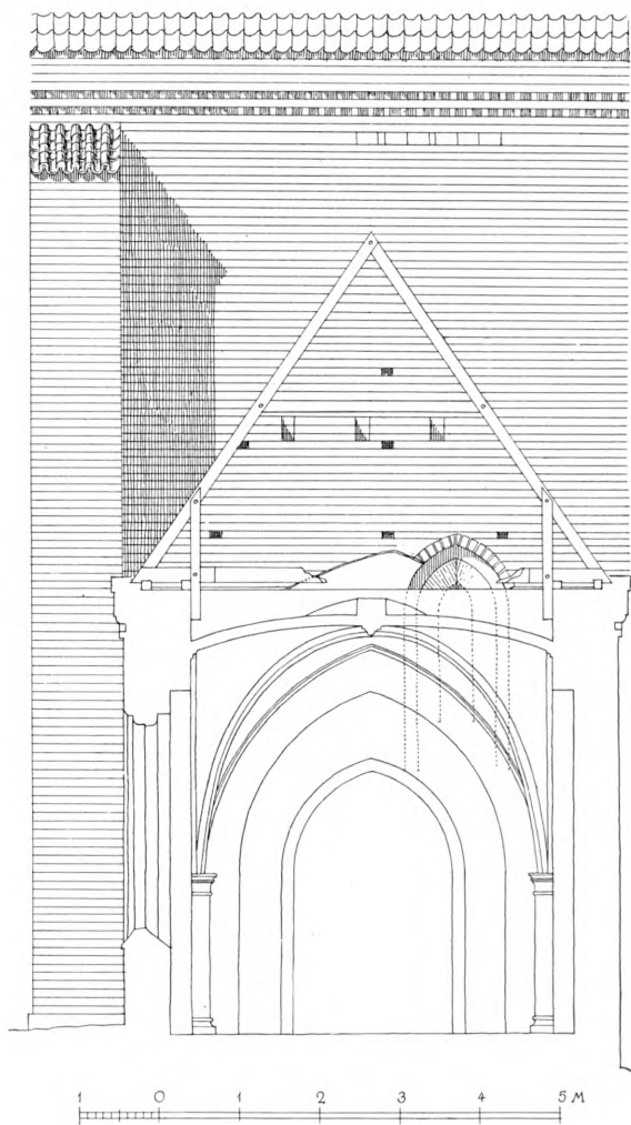
Fig. 2. Næstved S. Morten. Snit i nordre Vaabenhuse maalt af C. G. Schultz 1932.
