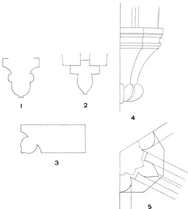
Fig. 4. Næstved S. Morten. Formstensprofiler, 1:10, maalt af C. G. Schultz 1932. 1. Hvælvingsribbe i Skibet. 2. i Koret. 3. Karm om Korets Syddør. 4—5. Hvælvingskonsol i Koret.
