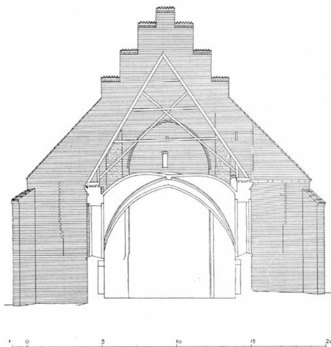
Fig. 4. Vordingborg. Skibets Østgavl og Snit af Koret. Maalt af C. G. Schultz 1932.
