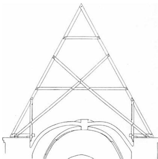
Fig. 5. Vordingborg. Sakristiets Tagværk. Maalt af C. C. Schultz 1932.
