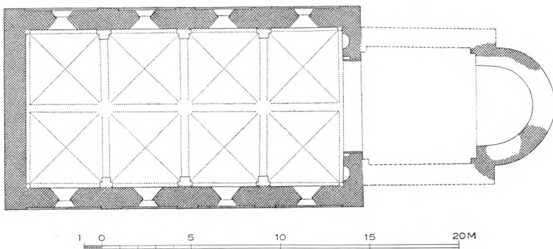
Fig. 4. Stege. Rekonstrueret Plan af den romanske Kirke (uden Taarne). Maalt af C. G. Schultz 1930.
