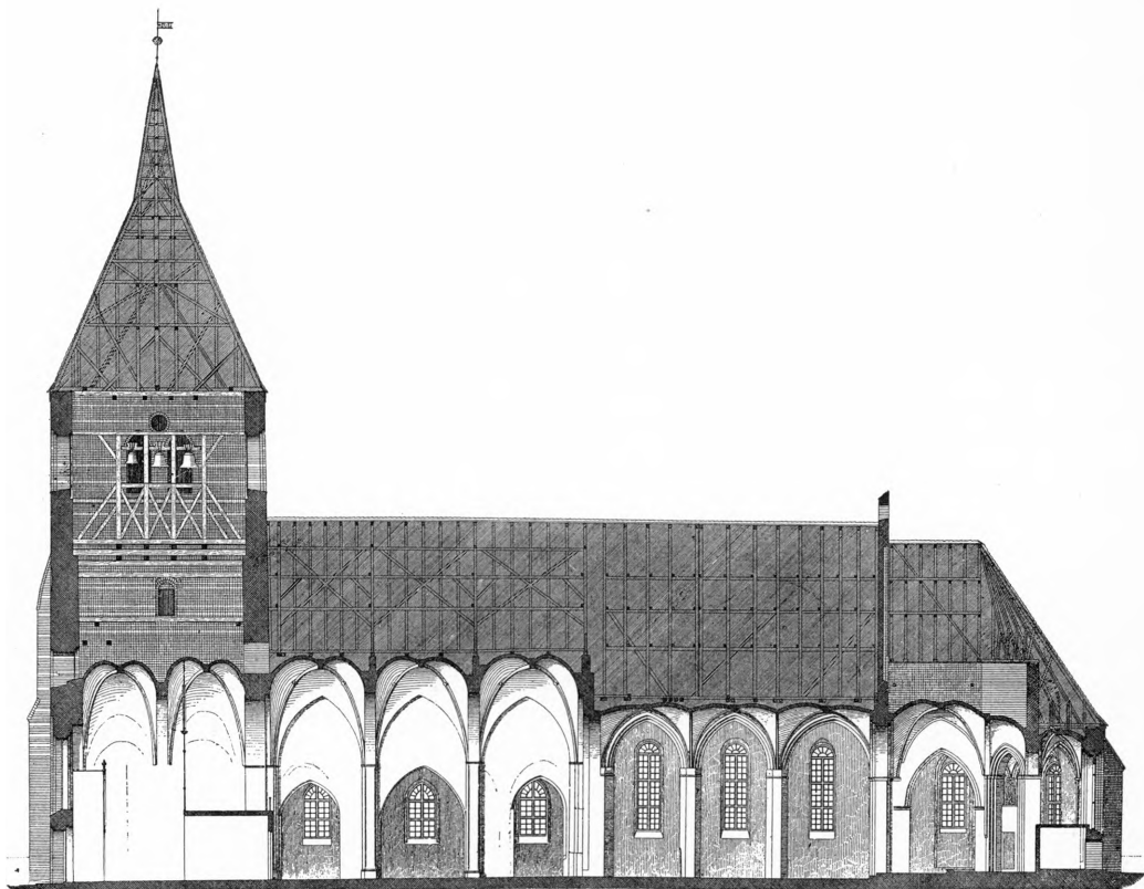
Fig. 8. Stege. Langsnit, set mod Nord. Efter Opmaaling 1902 i »Eldre nord. Architectur«.
