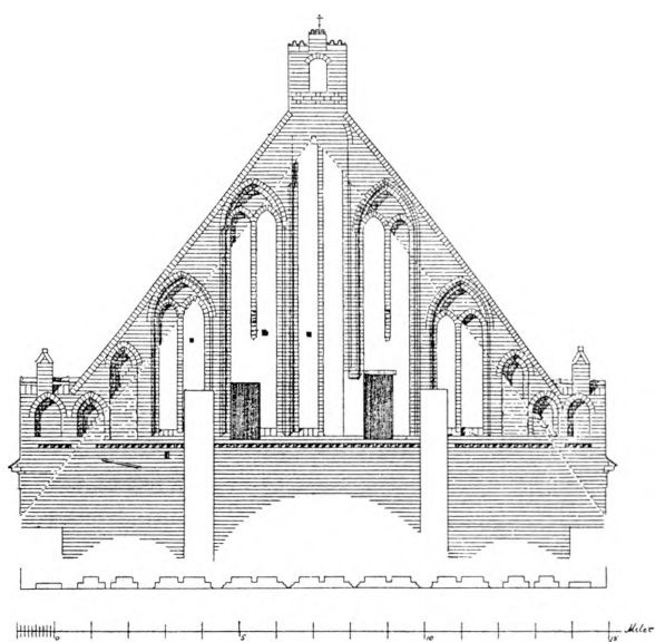
Fig. 6. Stege. Østgavlen paa det første gotiske Kor. Efter Opmaaling 1902 i »Eldre nord. Architectur«
