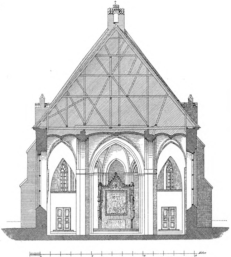
Fig. 7. Stege. Tværsnit af det første gotiske Kor, set mod Øst. Efter Opmaaling 1902 i »Eldre nord. Architectur«
