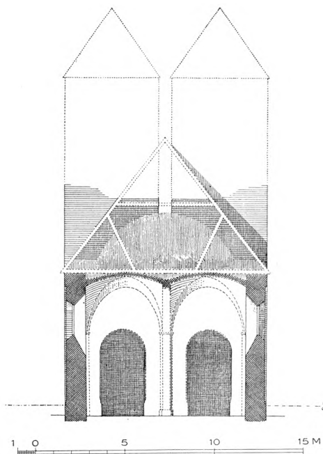
Fig. 3. Stege. Rekonstrueret Tværnit af den romanske Kirke, set mod Vest. Maalt af C. G. Schultz 1930.
