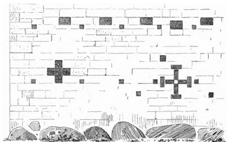
Fig. 3. Bjeverskov. Parti af Korgavlen. Op- maalt 1893 af V. Koch.
