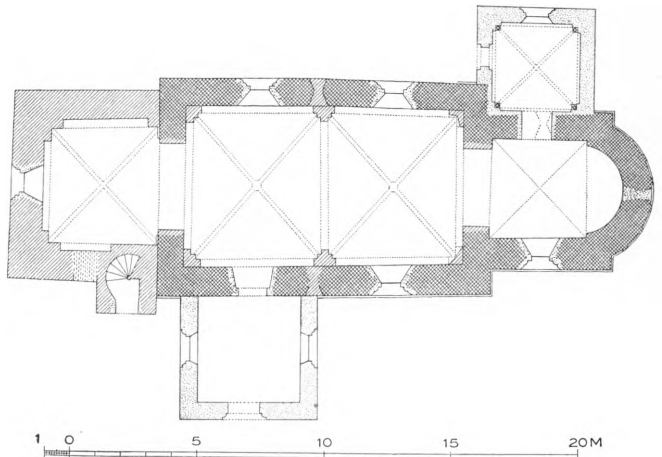
Fig. 2. Sædder. Plan. 1:300. Maalt af E. Schiødtte 1875, Otto Langballe 1927 (C. G. Schultz 1931).
