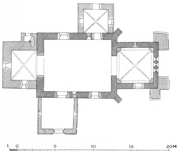
Fig. 4. Højerup. Plan. 1:300. Maalt af Helge Holm 1915 (C. G. Schultz 1932).
