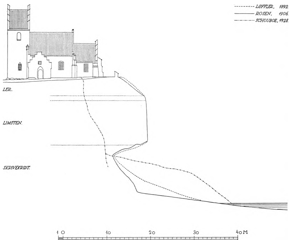
Fig. 3. Højerup. Snit, 1:500, af Klinten med Jordlag og Nedstyrtningslinier (C. G. Schultz 1932).
