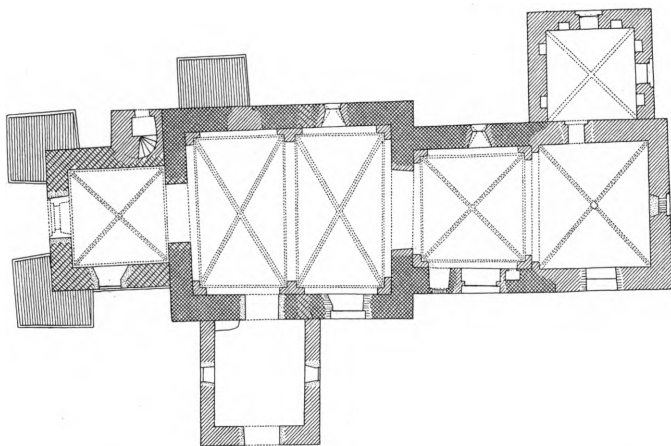
Fig. 2. Varpelev. Plan. 1:300. Maalt af Helge Holm 1915 (C. G. Schultz 1932).
