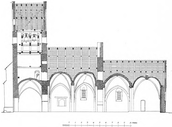
Fig. 4. Varpelev. Langsnit. 1:300. Maalt af Aage Sattrup og Johs. Kjær 1931. Taarnets tilmurede Glugger er ikke viste i Langsnittet.
