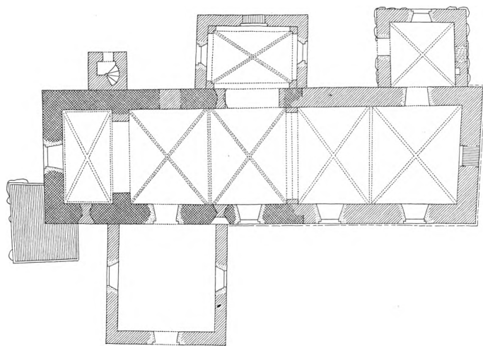
Fig. 2. Lyderslev. Plan. 1:300. Maalt af K. V. Barfoed 1914 (C. G. Schultz 1932).
