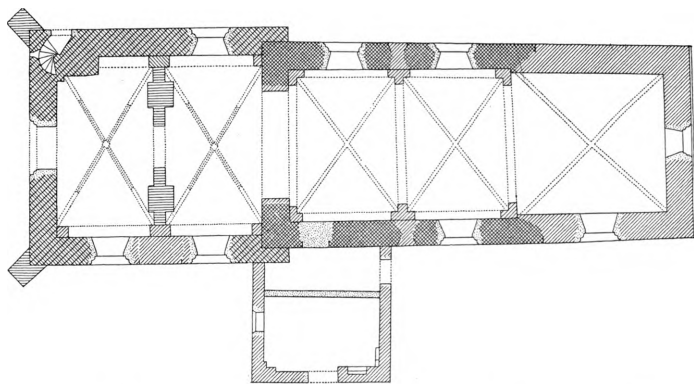
Fig. 2. Frøslev. Plan. 1:300. Maalt af Helge Holm 1915 (C. G. Schultz 1932).
