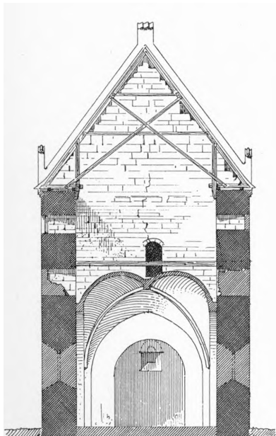
Fig. 5. Lillehedinge. Tværsnit, set mod Øst, af Skibet. 1: 200. Maalt af V. Koch 1894.
