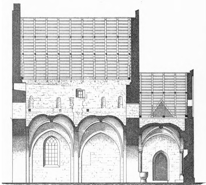
Fig. 6. Lillehedinge. Længdesnit, set mod Nord, af Skib og Kor. 1:200. Maalt af J. B. Løffler 1893. Det gotiske Taarn er udeladt.
