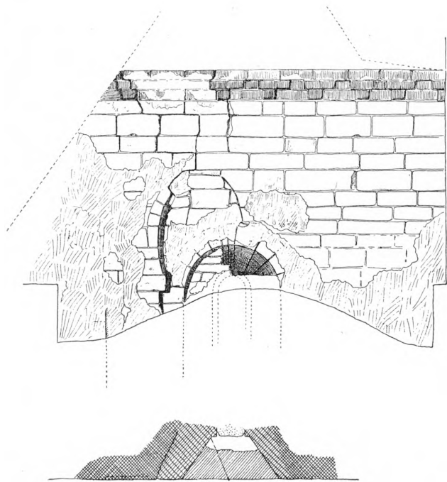
Fig. 3. Lillehedinge. Romanske Vinduer paa Korets Nordmur. 1:50. Maalt af K. V. Barfoed 1916.
