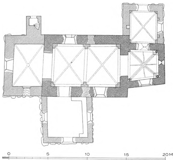
Fig. 2. Lillehedinge. Plan. 1:300. Maalt af Helge Holm 1915 (C. G. Schultz 1932).
