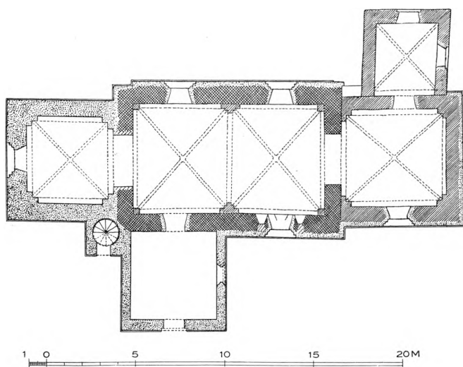
Fig. 2 Havnelev. Plan. 1:300. Maalt af Helge Holm 1915 (Charles Christensen 1932).
