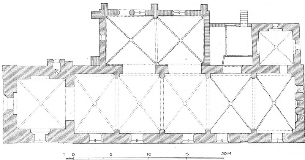
Fig. 2. Fakse. Plan. 1:300. Maalt af K. V. Barfoed 1914 (Aage Roussell 1930).
