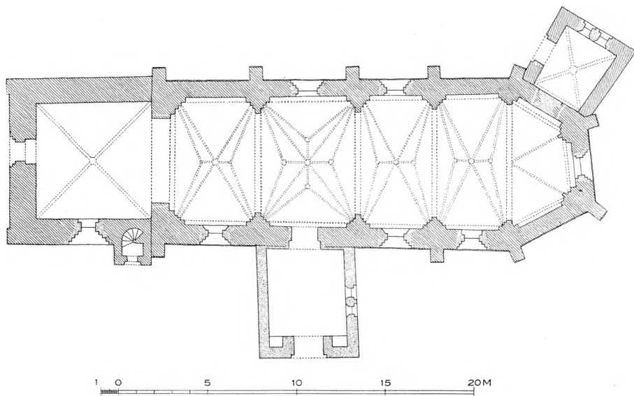
Fig. 2. Roholte. Plan. 1:300. Maalt af K. V. Barfoed 1914 (Aage Roussel 1929).
