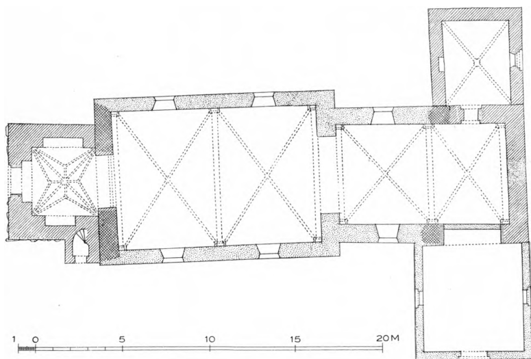
Fig. 2. Næsbjerg. Plan. 1:300. Maalt af Th. Havning 1917 (Aage Roussell 1930).
