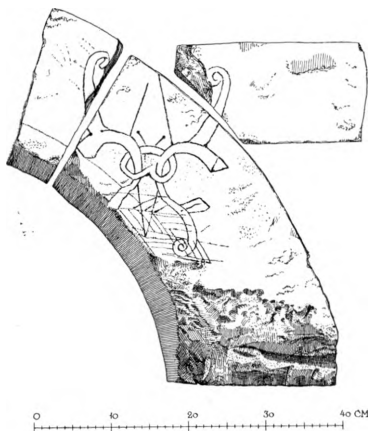
Fig. 4. Hammer. Korets Nordvindue. 1:10. Maalt af C. G. Schultz 1934.
