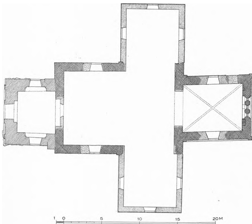
Fig. 2. Køng. Plan. 1:300. Maalt af Th. Havning 1917 (Aage Roussell 1930).
