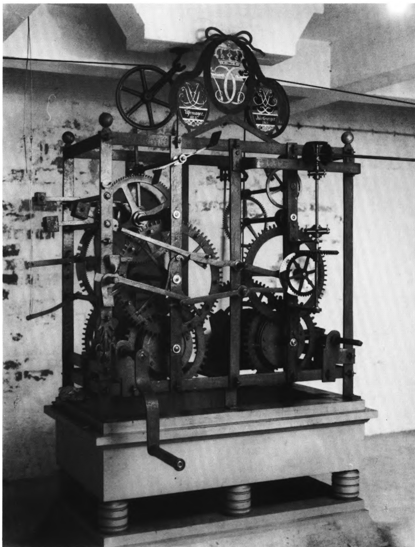
Fig. 80. Urværk, 1802, udført af urmager Jens Schultz (s. 770). NE fot. 1979. — Uhrwerk, 1802, ausgeführt von Uhrmacher Jens Schultz.
