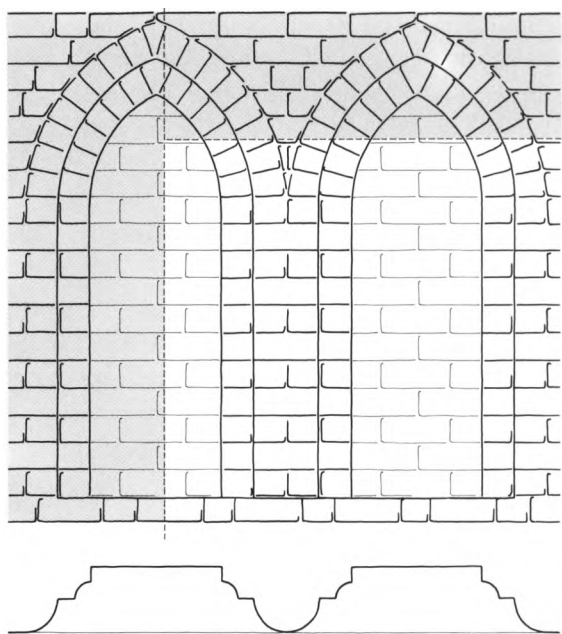
Fig. 15. Kirke nr. 2. Opmåling (og rekonstruktion) af delvis skjulte gavlblændinger (s. 702). 1:50. Målt af ELM, tegnet af MN 1983. — Kirche Nr. 2. Vermessung (und Rekonstruktion) teilweise verborgener Giebelblenden.
