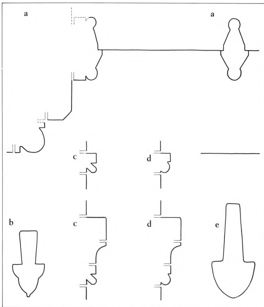
Fig. 26. Detaljer 1:10. a. Karm- og stavværksprofil i sydurens to østre vinduer (s. 708.) b. Ribbesten fra nordre sideskib (s. 711). c. Kragbånd og kordongesims i kirkens to østre fag. d. Samme i kirkens fire vestre fag (s. 708). e. Ribbesten (fra kirke nr. 1-2?), fundet to meter under korgulvet (s. 701). Efter Axel Hansen og C. M. Smidt. Tegnet af MN 1984. — Details. 1:10. a. Rahmen- und Stabwerkprofil der zwei östlichen Fenster in der Südwand, b. Rippenstein aus dem nördlichen Seitenschiff, c. Kragsteine und Kordonsimse in den zwei östlichen Fächern der Kirche, d. Dasselbe in den vier westlichen, e. Rippensteine (aus der Kirche Nr. 1-2?), gefunden zwei Meter unter dem Fußboden des Chors.
