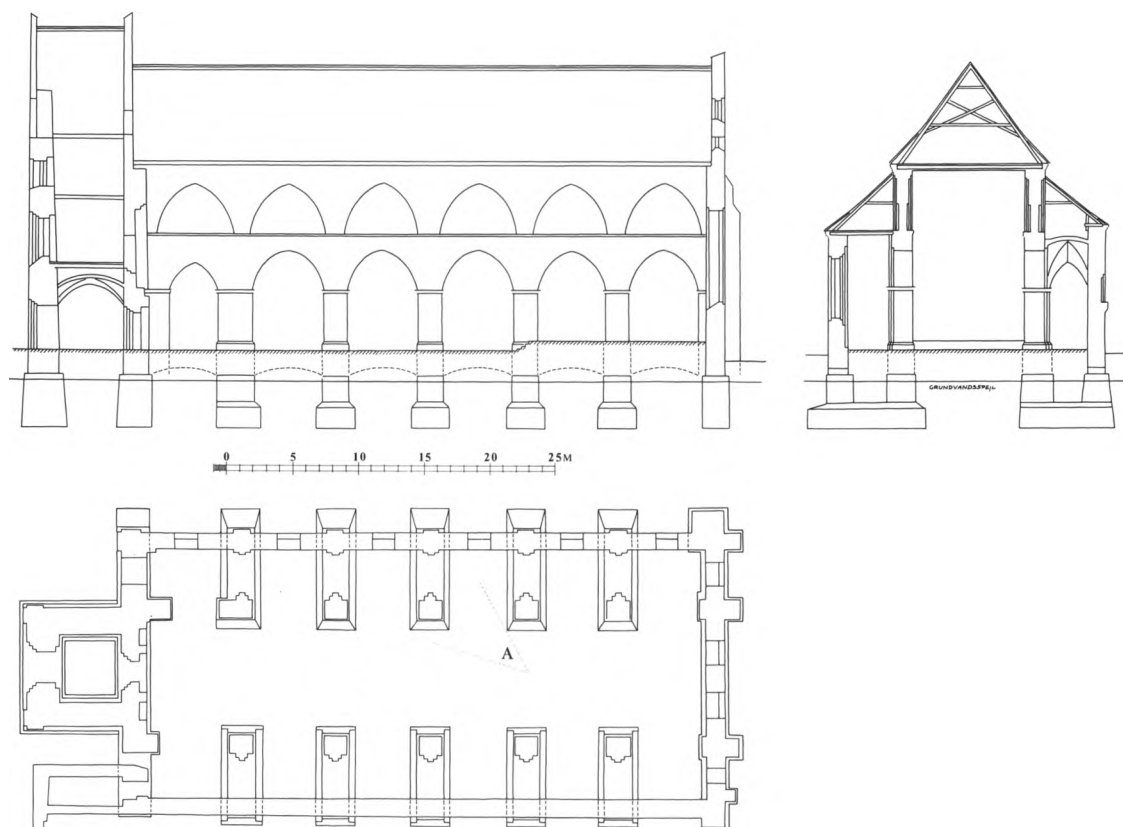
Fig. 35. Kirkens nyfundering 1918-19 (s. 720). Plan og snit. 1:600. Efter G. Schönweller, tegnet af MN 1983. (A markerer fotograferingsvinklen for fig. 36). — Neufundamentierung der Kirche 1918-19. Grundriß und Schnitt. 1:600. (A bezeichnet den Aufnahmewinkel für Fig. 36).
