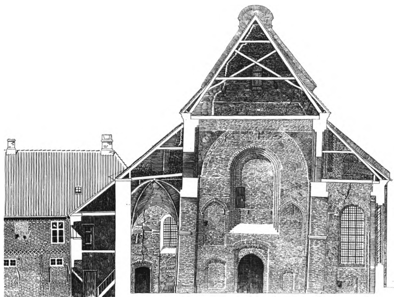
Fig. 24. Tværsnit, set mod vest. 1:300. Efter Axel Hansen 1918 f. — Querschnitt, gegen Westen gesehen.
