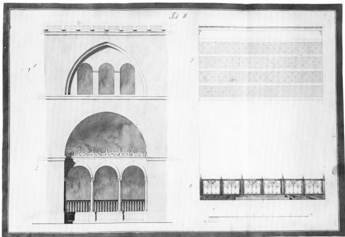
Fig. 67. Theophilus Hansens farvelagte tegning (Tab. II) med forslag til kirkens forskønnelse 1837. Tallene angiver: 1 Opstalt af midtskibet mod syd (s. 716); gennem arkaden ses pulpitur (2) i søndre sideskib (†nr. 2, s. 760). 3 Bemaling af midtskibets træloft, lyseblåt med stjerner (s. 731). 4 Korgitter af træ (†nr. 3, s. 749). I LA Vib. — Theophil Hansens ausgemalte Zeichnung (Tab. II) mit Vorschlägen zur Verschönerung der Kirche, 1837. Die Ziffern bedeuten: 1. Aufriß des Mittelschiffs nach Süden gesehen; durch die Arkade sieht man die Empore (2) im südlichen Seitenschiff. 3. Bemalung der Holzdecke des Mittelschiffs, hellblau mit Sternen. 4. Chorgitter aus Holz.
