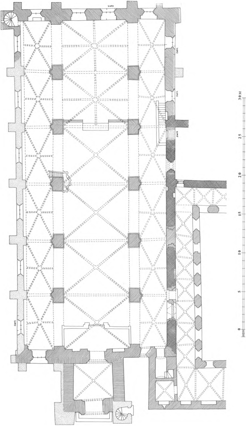
Fig. 13. Plan. 1:300. Øst opad. Målt af Axel Hansen 1918f. Suppleret af EIM, tegnet af MN 1983. — Grundriß 1:300. Vermessen von Axel Hansen 1918f., ergänzt von EIM.
