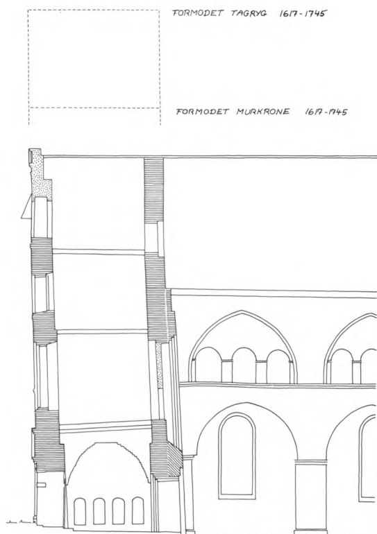
Fig. 41 a-c. Tårnet fra 1617-18. 1:300. a. Tværsnit set mod nord. Efter opmåling af Axel Hansen 1918. b-c. Tværsnit set mod nord og vest. Efter Lønborg Jensen 1925. Tegnet af MN 1983. — a-c. Der Turm von 1617-18. 1:300. a. Querschnitt gegen Norden gesehen. b.-c. Querschnitt gegen Norden und Westen gesehen.
