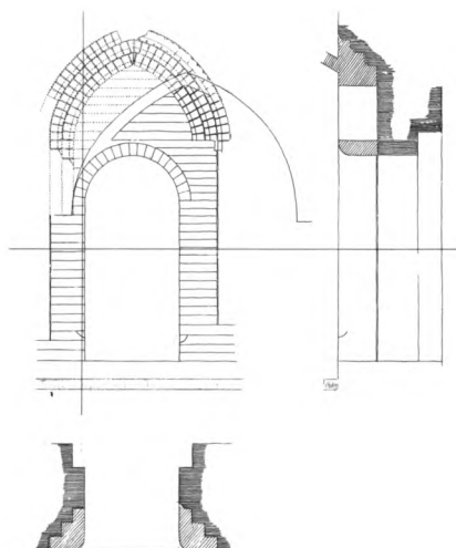
Fig. 17. Kirke nr. 2. Spidsbuet, falset dør til klostergården. Omdannet og delvis dækket ved opførelsen af nordre korsgang (s. 708). 1:100. Efter Axel Hansen, 1924. — Kirche Nr. 2. Spitzbogige, gefälzte Tür zum Klosterhof. Umgestaltet und teilweise gedeckt bei der Aufführung des nördlichen Kreuzgangs.
