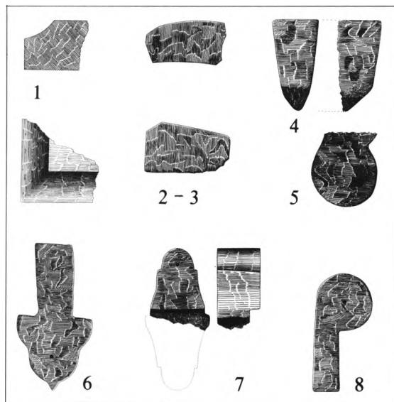
Fig. 8. S. Klemens kirke. Formsten. 1. Sokkelled med hulkel af tuf (s. 833). 2. Fragment af buesten, tuf (s. 835). 3. Profileret tufsten (s. 835). 4. Konsol af tuf (s. 835). 5. Trekvartsøjleled af tuf (s. 833). 6. Ribsten fra skibets vestvæg. 7. Stein aus Stabwerk, Ziegel. 8. Rundstab aus Ziegel.
