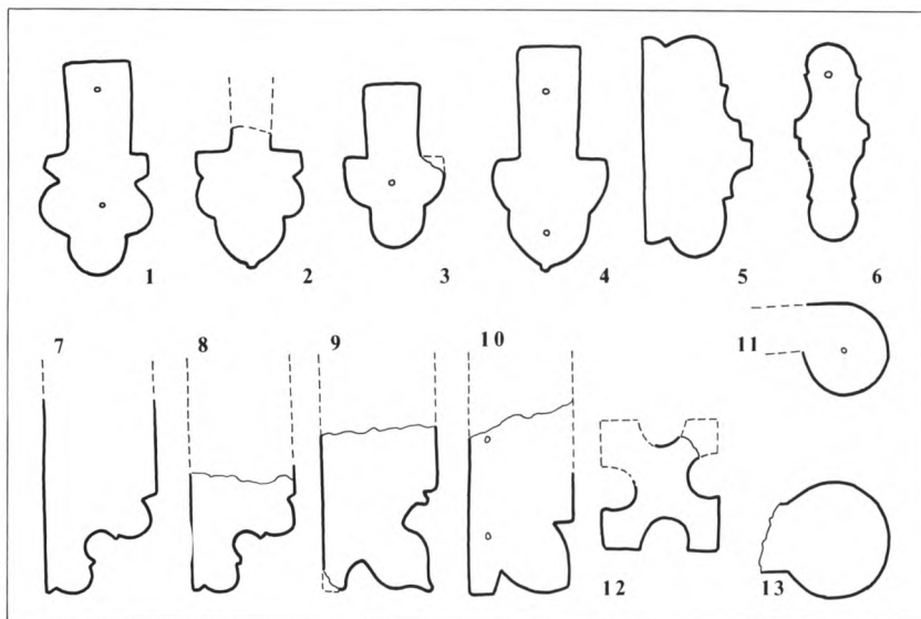
Fig. 20. Franciskanerklostret. Formsten af tegl (s. 848). 1-4. Ribbesten. 5-6. Vinduesstadværk. 7-13. Andre profilsten (12 fra kløverbladsfrise, 13 fra spindeltrappe?). 1:10. Målt af ELM, tegnet af MN 1984. — Franziskanerkloster. Formsteine aus Ziegel. 1-4. Rippensteine, 5-6. Fensterstabwerk. 7-13. Andere Profilsteine (12 aus einem Kleeblattfries, 13 von einer Spindeltrappe?) .
