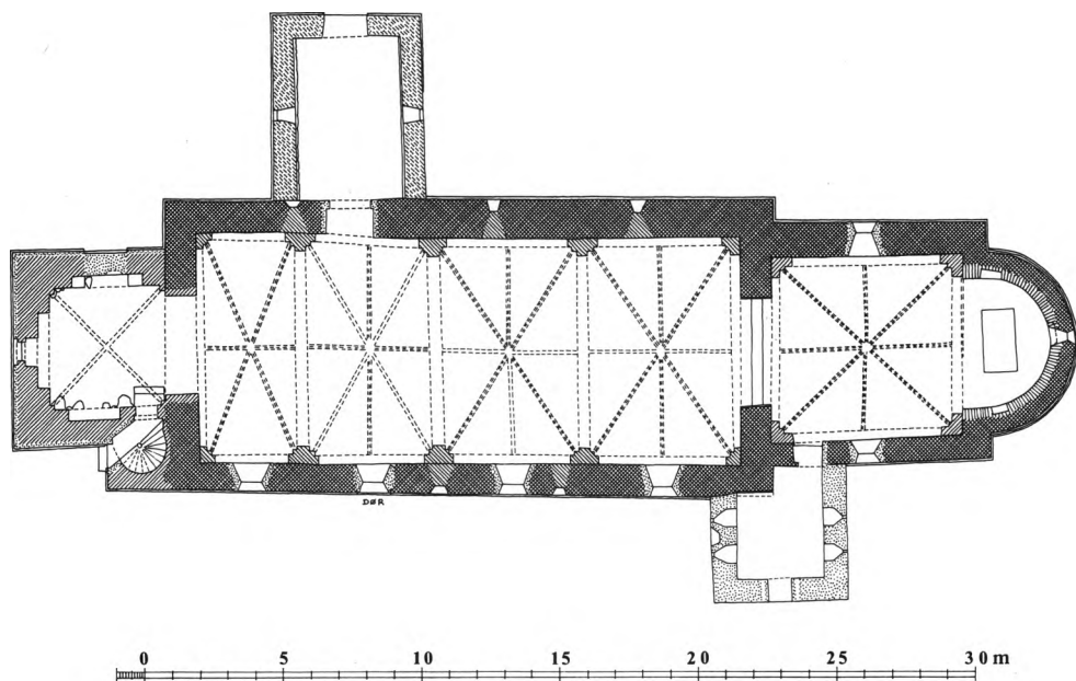
Fig. 4-5. Grundplan 1:300 og tværsnit 1:150 gennem skib. Målt af Henrik Gram og Søren Gottfred Petersen 1978, tegnet af MN 1985. — Grundriß 1:300 und Querschnitt 1:150 durch das Schiff.
