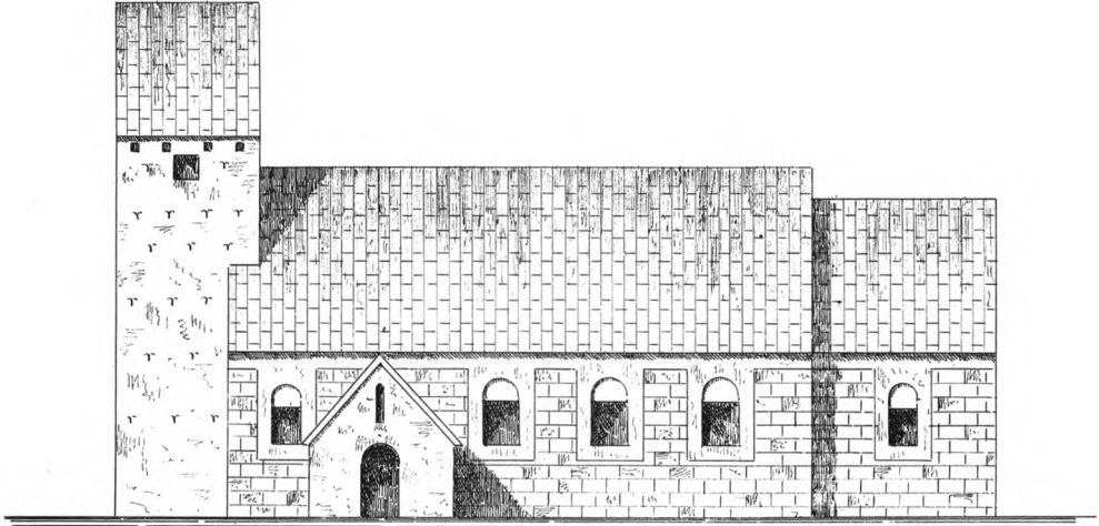
Fig. 4. Kirkens sydside 1:300, målt og tegnet af L. A. Winstrup o. 1876. — Die Südseite der Kirche 1:300, vermessen und gezeichnet um 1876.
