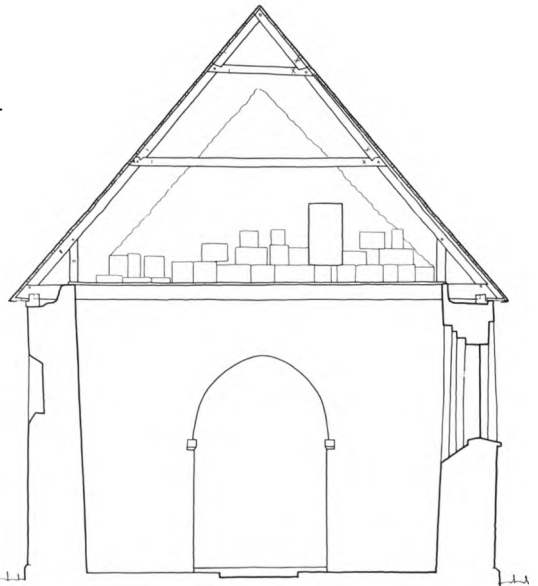
Fig. 5. Tværsnit 1:150 gennem skib, set mod øst. Målt af Henrik Gram og Søren Gottfred Petersen 1979 og tegnet af MN 1985. — Querschnitt 1:150 durch das Schiff, gegen Osten gesehen.
