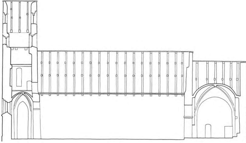
Fig. 2. Længdesnit 1:300 gennem skib, set mod nord. Målt af arkitekterne Aas og Thorup 1980, tegnet af MN 1985. — Längsschnitt 1:300 durch das Schiff, gegen Norden gesehen.
