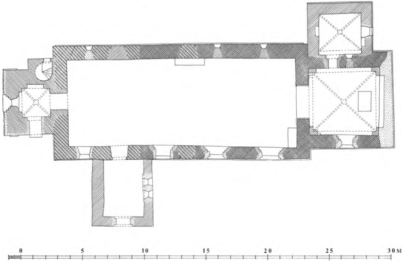
Fig. 3. Grundplan 1:300. Målt af Henrik Gram og Søren Gottfred Petersen 1979 med enkelte rettelser ved NJP. Tegnet af MN 1985. — Grundriß 1:300.
