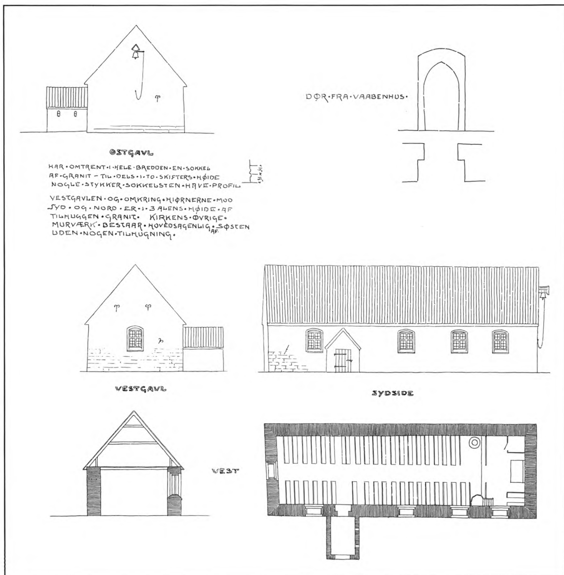
Fig. 7. Plan, snit og opstalter af den gamle kirke, 1:300, samt detalje af syddøren, 1:100, målt og tegnet af J. Magdahl Nielsen i juli 1903, kort før kirkens nedrivning. NM2. — Grundriss, Schnitt und Aufrisse der alten Kirche, 1:300, sowie Detail der Südtür, 1:100. Zeichnung 1903, kurz vor Abbruch der Kirche.
