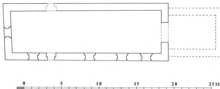
Fig. 4. Grundplan 1:300 af den nedrevne Ækirke forud for korets nedbrydning og våbenhusets tilkomst 1750. Korets omtrentlige længde, men ikke bredden, er kendt. Om norddøren vides det kun, at den sad over for syddøren. Rekonstruktionsforslag på grundlag af fig. 7, tegnet af NJP og MN 1986. — Grundriss 1:300 der niedergerissenen ÆKirche vor Abbruch des Chors 1750 und Errichtung der Vorhalle. Die Länge, nicht aber die Breite des Chors ist bekannt. Von der Nordtür weiss man nur, dass sie gegenüber der Südtür war. Zeichnung 1986.
