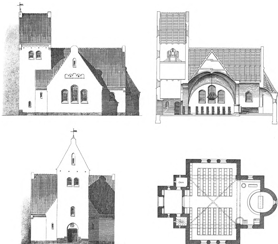
Fig. 2. Lønne nye kirke. Plan, snit og opstalter 1:300. Tegninger publiceret af arkitekt J. Magdahl Nielsen i Arkitekten 1904. — Neue Kirche von Lønne. Grundriss, Schnitt und Aufrisse 1:300. Zeichnungen 1904.
