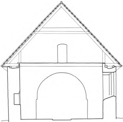
Fig. 3-4. Grundplan 1:300 og tværsnit 1:150 gennem skib, set mod øst. Målt af HeJ og NJP i marts 1985, tegnet af MN 1987. — Grundriss 1:300 und Querschnitt 1:150 durch das Schiff, gegen Osten gesehen.
