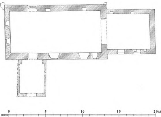
Fig. 3-4. Grundplan 1:300 og tværsnit 1:150 gennem skib, set mod øst. Målt af HeJ og NJP i marts 1985, tegnet af MN 1987. — Grundriss 1:300 und Querschnitt 1:150 durch das Schiff, gegen Osten gesehen.
