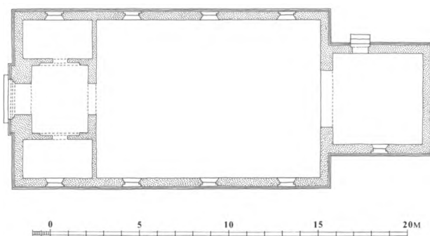
Fig. 3. Grundplan 1:300 af Oksby ny kirke. Udkast af F. Uldall 1889, omtegnet af M. Nielsen 1987. Blåvandshuk lokalhistoriske arkiv. — Grundriss 1:300 der neuen Kirche von Oksby. Entwurf 1889, umgezeichnet 1987.
