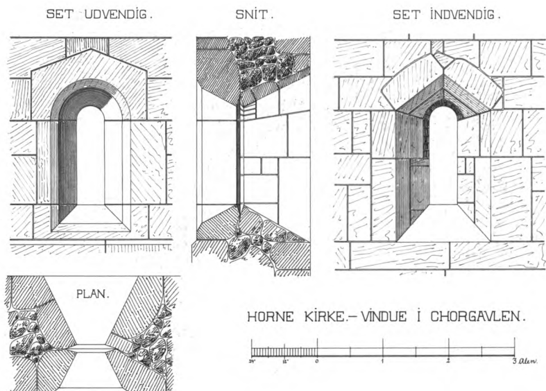
Fig. 5. Plan, snit og opstalter 1:50 af romansk vindue i korets østgavl (s. 1446). Målt og tegnet af Hector Estrup 1887.
