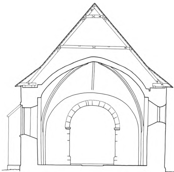
Fig. 4. Tværnsnit 1:150 gennem skib, set mod øst. Målt af Henrik Gram og Søren Gottfred Petersen 1979. Tegnet af MN 1987. — Querschnitt durch das Schiff nach Osten .
