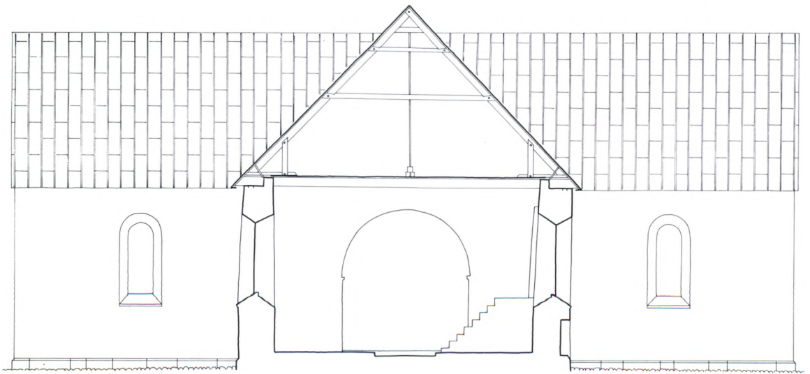
Fig. 4. Tværsnit 1:150 gennem skibets vestende set mod øst. Målt af Henrik Gram og Søren Gottfred Petersen 1981. Tegnet af MN 1988. – Querschnitt durch Westteil des Schiffs nach Osten .
