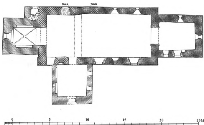
Fig. 2. Grundplan 1:300. Målt af Henrik Jacobsen 1983. Tegnet af Marianne Nielsen 1989. – Grundriss.
