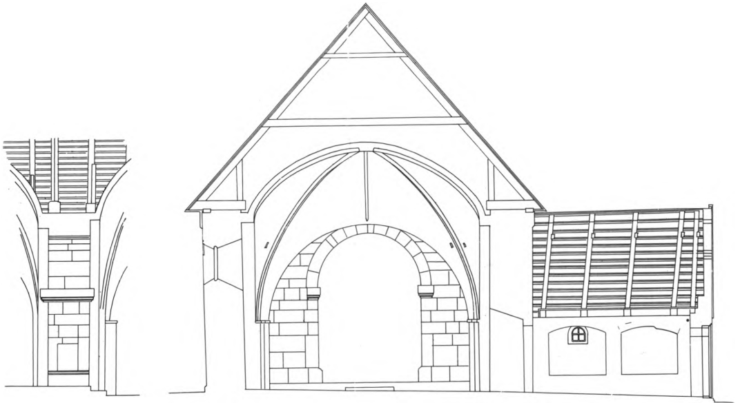
Fig. 8-9. Snit gennem kirken, 1:150, målt og tegnet af Hector Estrup 1890. 8. Snit gennem triumfbue, set mod syd. 9. Tværsnit gennem skib og † våbenhus, set mod øst. – 8. Schnitt durch Triumphbogen gegen Süden. 9. Querschnitt durch Schiff und † Vorhalle gegen Osten. 1890.
