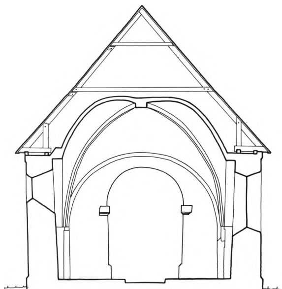
Fig. 4. Tværsnit 1:150 gennem skib, set mod øst. Målt af Henrik Jacobsen 1986, tegnet af Marianne Nielsen 1989. – Querschnitt durch Schiff nach Osten.
