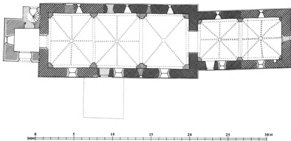
Fig. 3. Grundplan 1:300. Målt af Henrik Jacobsen 1986, tegnet af Marianne Nielsen 1989. – Grundriss.
