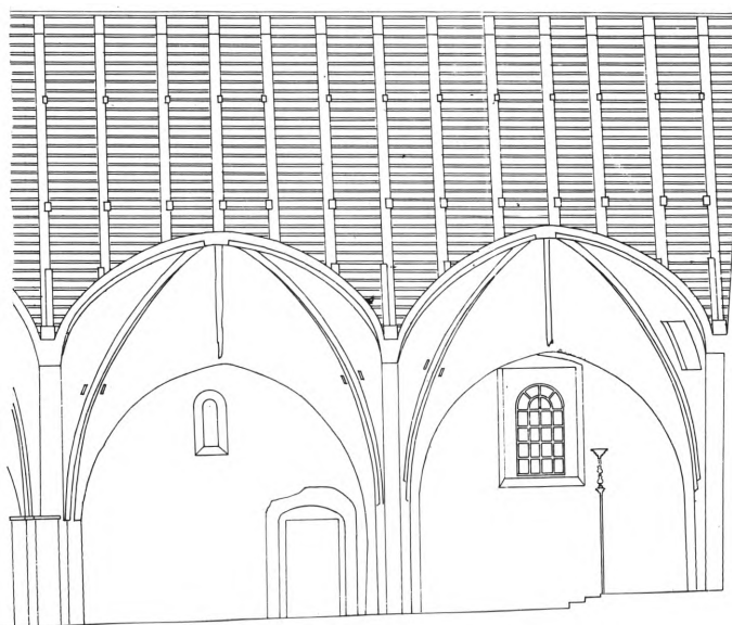
Fig. 10. Længdesnit gennem skibets to vestre hvælvfag, set mod syd, 1:150, målt og tegnet af Hector Estrup 1890. Det hævdede parti vestligst i skibet rummede en åben † begravelse, adskilt fra kirken ved et rækværk (s. 1907). – Längsschnitt nach Süden durch die zwei Westjoche des Schiffes . 1890.
