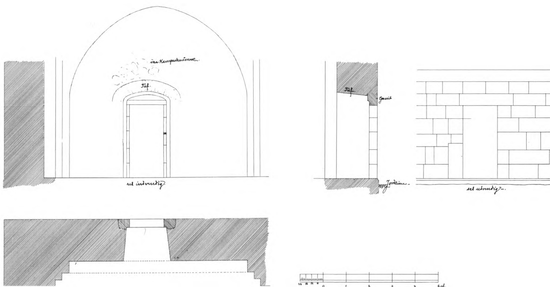
Fig. 35. Plan, opstalter og snit, 1:100, af tilmuret dør i vestforlængelsens nordside (s. 1884), målt og tegnet af Hector Estrup 1890. – Grundriss, Aufrisse und Schnitt einer vermauerten Tür in der Nordwand der Westverlängerung.
