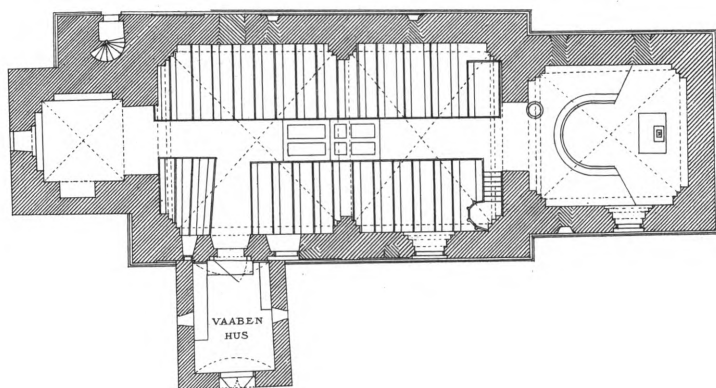
Fig. 31. Grundplan 1:300, målt og tegnet af V. Koch 1885. Efter Danske Tufstenskirkker. – Grundriss , 1885.
