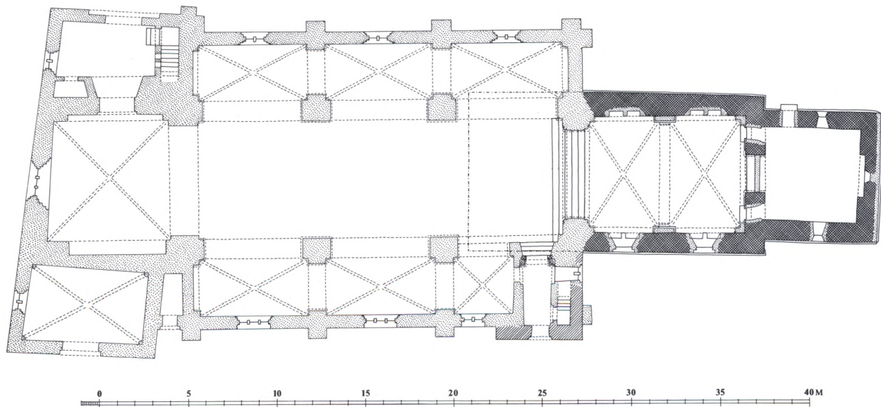
Fig. 8. Grundplan 1:300. Tegnet af Marianne Nielsen 1991 på grundlag af plan ved C. M. Smidt og Harald Lønborg-Jensen 1920 og opmåling af kirkens ældre dele ved Henrik Jacobsen 1986. De stiplede linier angiver den gamle kirkes udstrækning mod vest før udvidelsen. – Grundriss. Die punktierten Linien zeigen die Ausdehnung der alten Kirche vor der Erweiterung.
