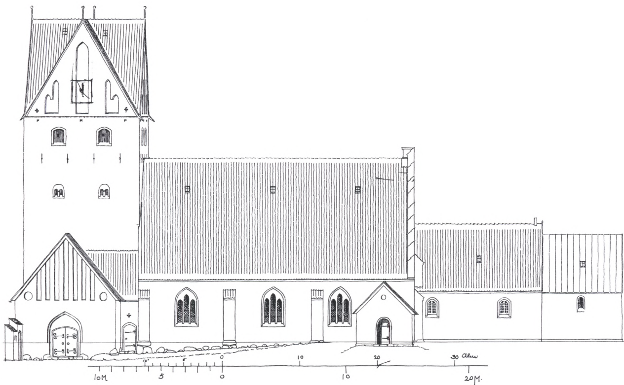
Fig. 7. Forslag til kirkens udvidelse. Opstalt af kirkens sydside, tegnet af Harald Lønborg-Jensen 1920. I Grindsted Museum. 1:300. – Vorschlag zum Ausbau der Kirche. Aufriss von der Südseite 1920.
