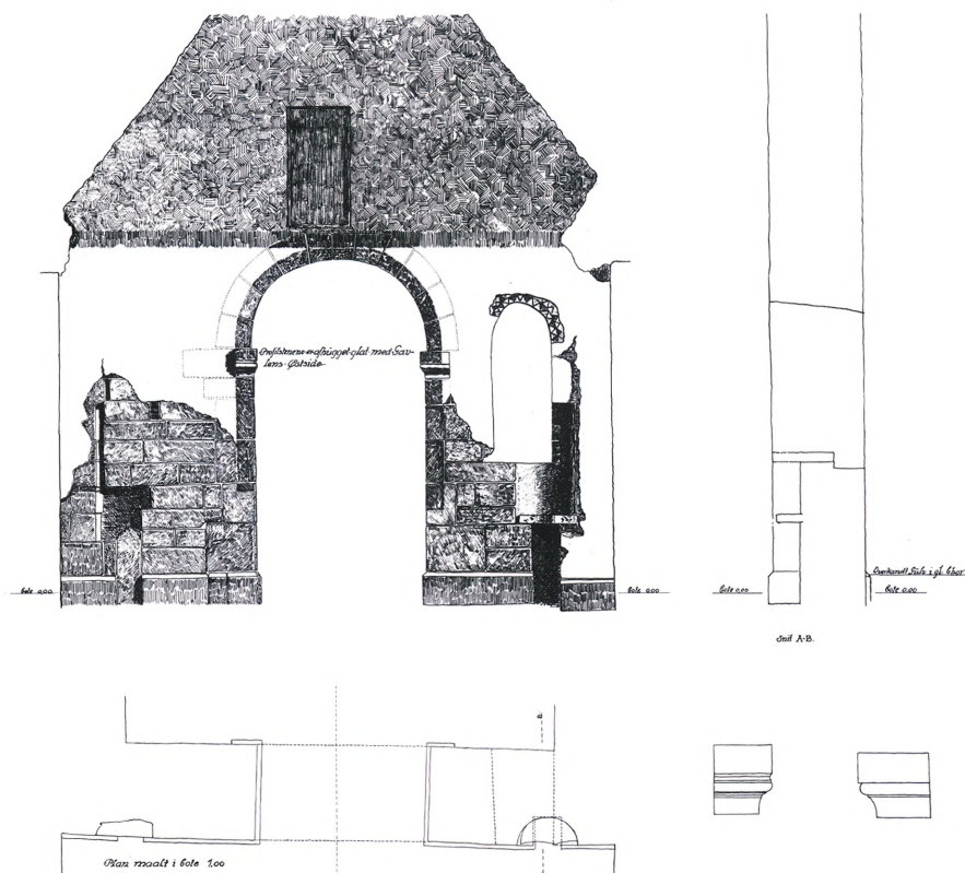
Fig. 15. Opmåling af triumfmuren (s. 2232) ved Harald Lønborg-Jensen 1920: vestside, plan og tværsnit. Den søndre sidealterniche er ødelagt ved gennembrydningen af en opgang til prædikestolen. 1:100. I NM. – Triumphwand: Westseite, Grundriss und Querschnitt. Vermessen 1920.
