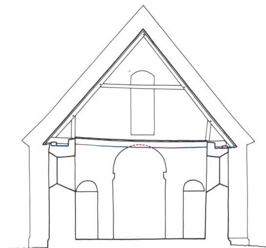
Fig. 14. Tværsnit 1:150 gennem koret, set mod vest. Målt af Henrik Jacobsen 1986, tegnet af Marianne Nielsen 1991. – Querschnitt durch Chor gegen Westen.
