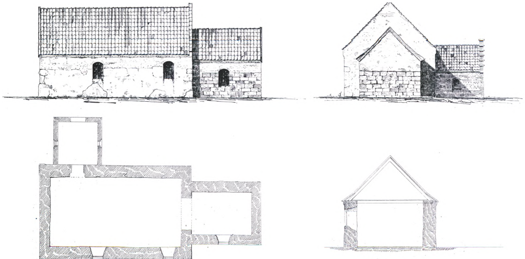
Fig. 4. Grundplan og tværsnit af skib, set mod vest, samt opstalter af kirkens syd og østside, målt og tegnet af J. Chr. Fussing 1887. 1:300. – Grundriss und Querschnitt von Schiff gegen Westen einschliesslich Aufrisse der Süd- und Ostseite der Kirche, 1887.
