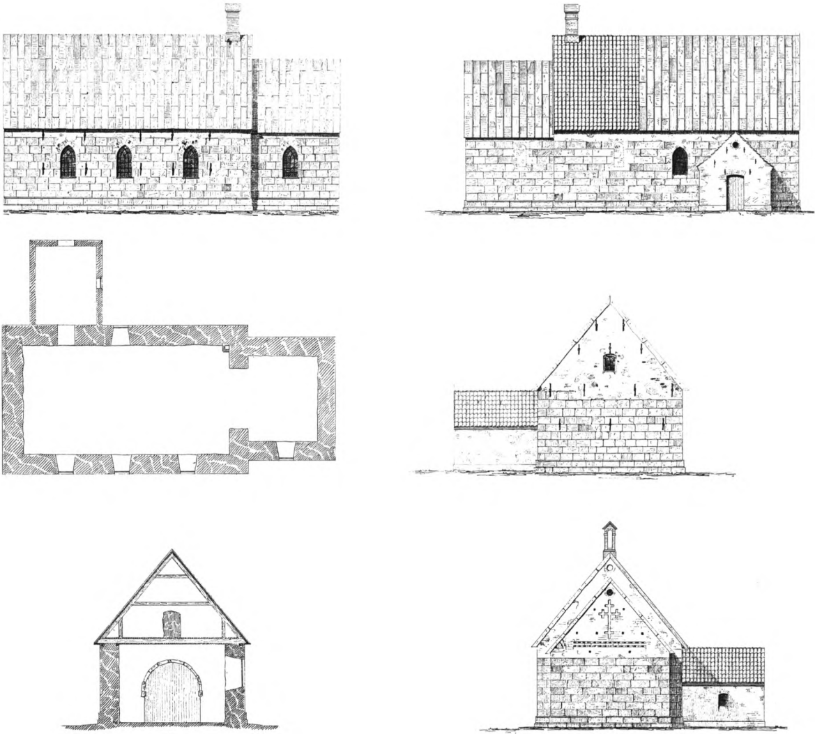
Fig. 2. Opstalter, grundplan og tværsnit gennem skib 1:300. Målt og tegnet af J. Chr. Fussing o. 1896. – Aufresse, Grundriss und Querschnitt durch Schiff.
