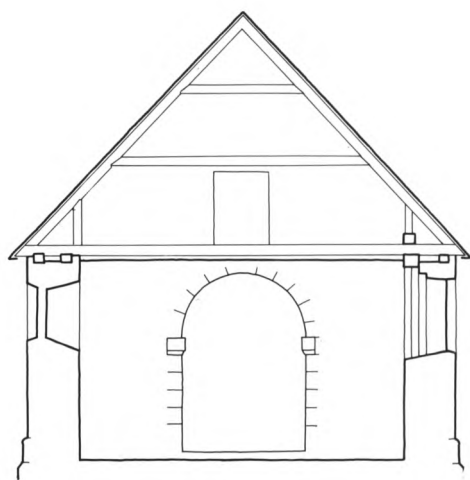
Fig. 6. Tværsnit gennem skib set mod øst, 1:150. Tegnet af Marianne Nielsen 1991 efter opmåling af Rud. Gram 1969. – Querschnitt durch Schiff gegen Osten.
