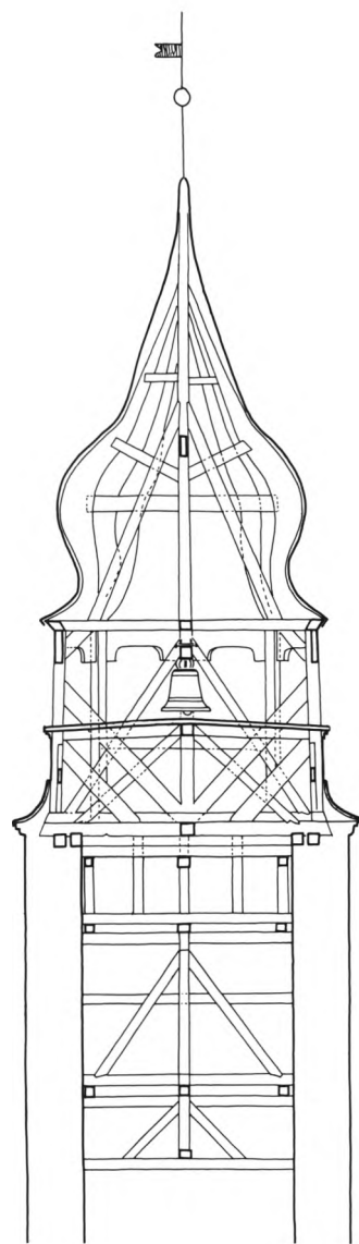
Fig. 21. Tårnets tagkonstruktion (s. 2476), målt af Harald Lønborg-Jensen 1942, tegnet af Marianne Nielsen 1992. 1:150. – Turm. Dachkonstruktion.
