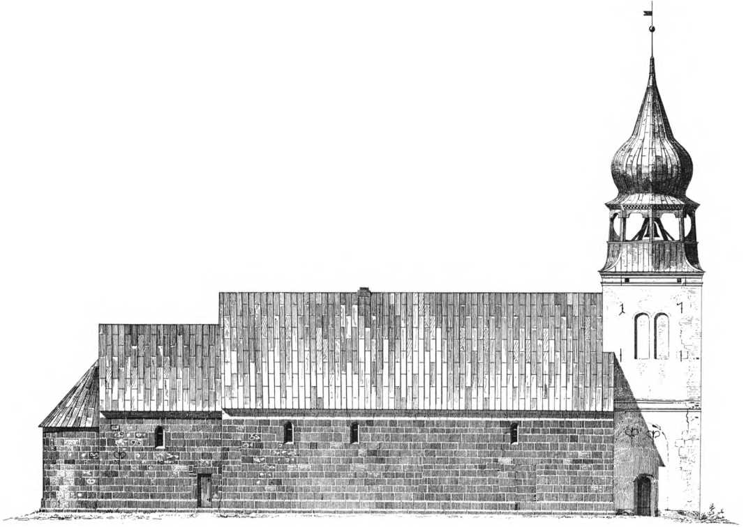
Fig. 5. Kirkens nordside 1:300, målt og tegnet af V. Koch 1892. Efter Jydske Granitkirker. – Nordseite der Kirche , 1892.
