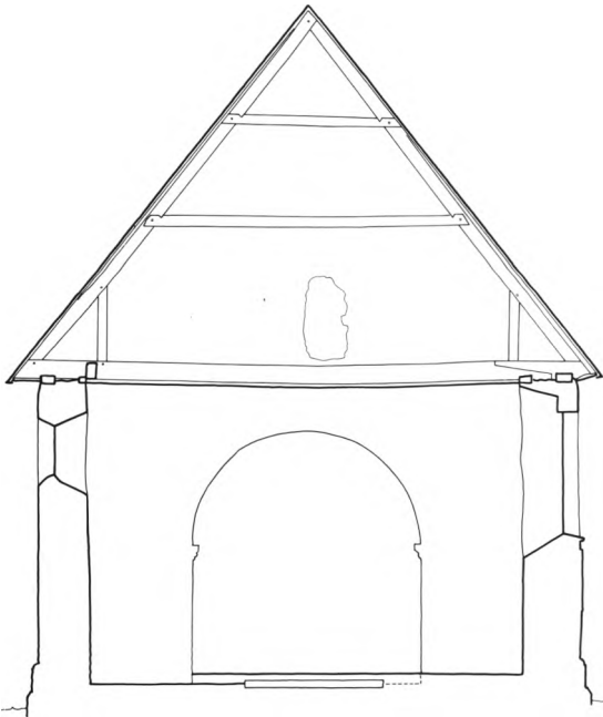
Fig. 19. Tværsnit 1:150 gennem skib, set mod øst. Målt af Henrik Jacobsen og tegnet af Marianne Nielsen 1992. – Querschnitt durch Schiff gegen Osten .
