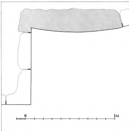
Fig. 8. Sammenstødet mellem apsis og kor, sydsiden. Målt af Henrik Jacobsen, tegnet af Marianne Nielsen 1992. – Verbindung zwischen Apsis und Chor, Südseite .
