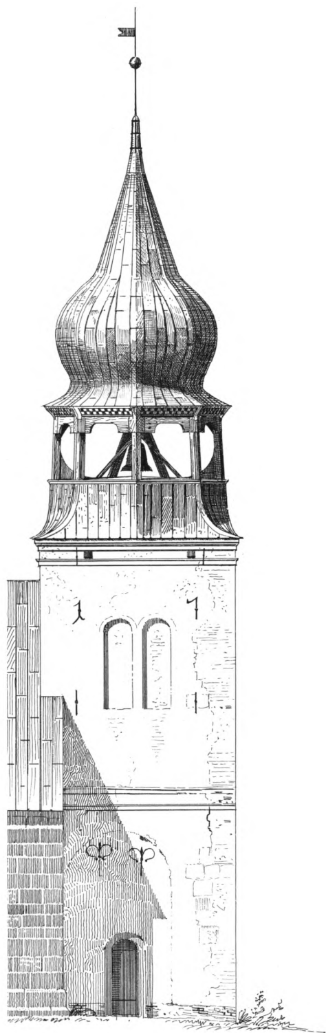
Fig. 20. Tårnet set fra nord. Målt og tegnet af V. Koch 1892. 1:150. Efter Jydske Granitkirker. – Turm. Nordansicht, 1892.
