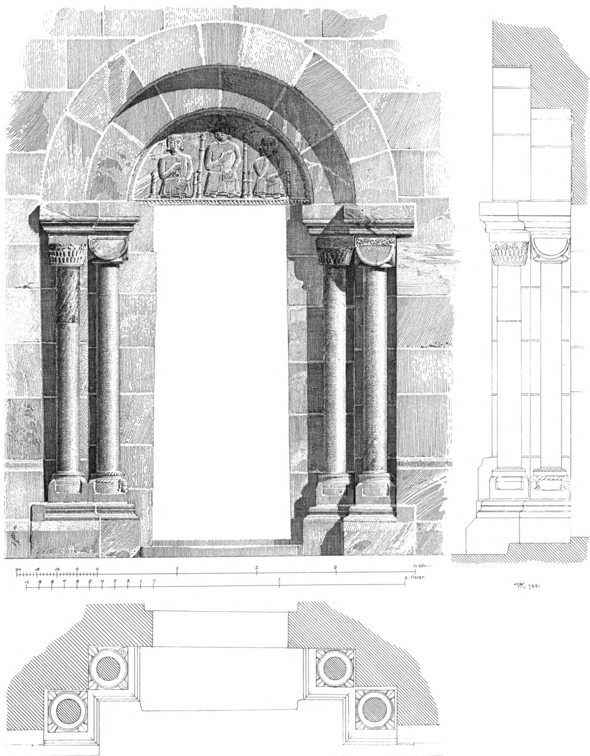
Fig. 12. Skibets sydportal. Opstalt, plan og snit (s. 2470). Målt og tegnet af V. Koch 1891. Efter Jydske Granitkirker. – Säulenportal in Schiffssüdwand. Aufriss, Grundriss und Schnitt, 1891.
