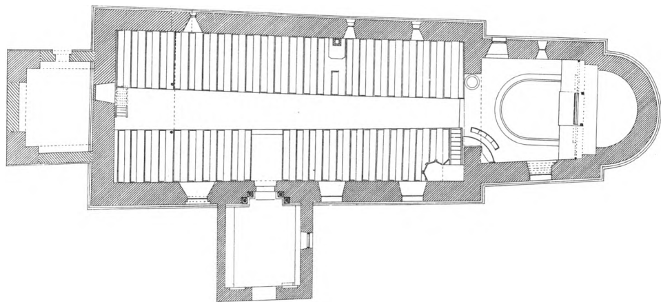
Fig. 22. Grundplan 1:300, målt og tegnet af V. Koch 1892. Efter Jydske Granitkirker. – Grundriss, 1892.
