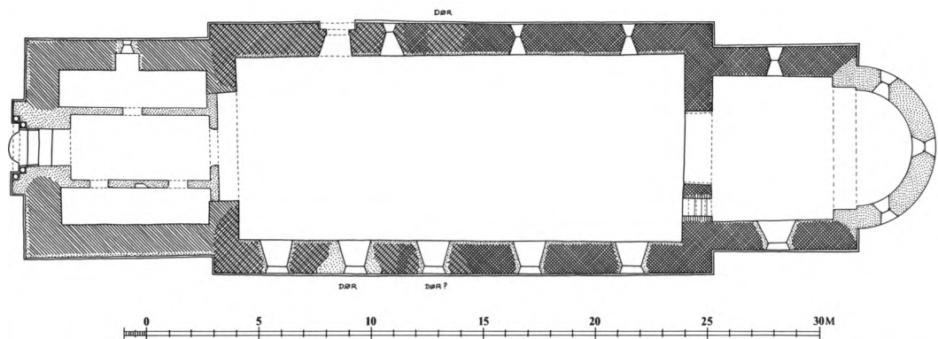
Fig. 4. Grundplan 1:300. Målt af Henrik Jacobsen 1988, tegnet af Marianne Nielsen 1992. – Grundriss.
