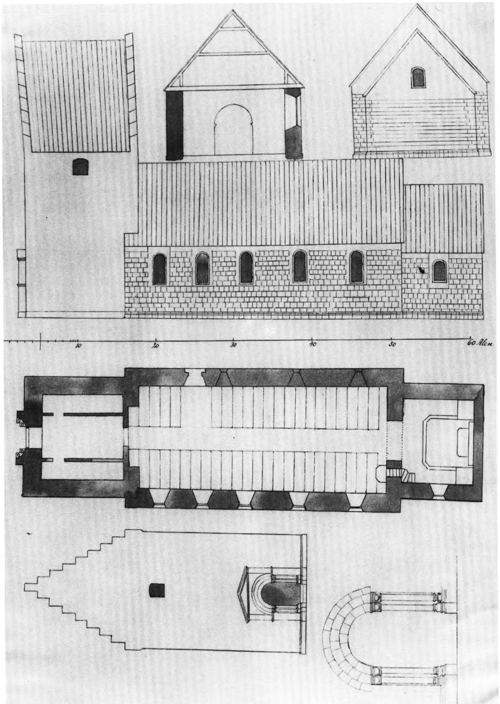
Fig. 16. Plan, snit og opstalter af kirken før ombygningen 1871-73. Tegning af G. Burman Becker 1870. Det kgl Bibliotek. – Grundriss, Schnitt und Aufrisse vor dem Umbau der Kirche 1871-73.
